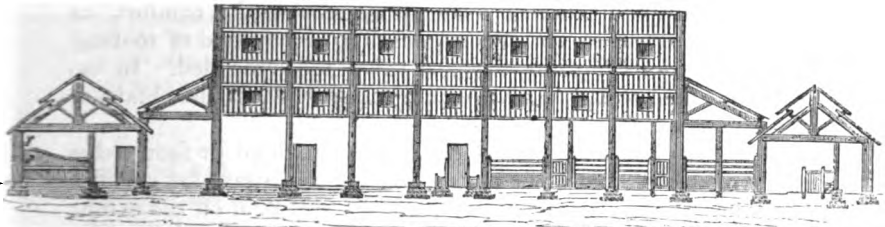
LONGITUDINAL SECTION—C. D.
