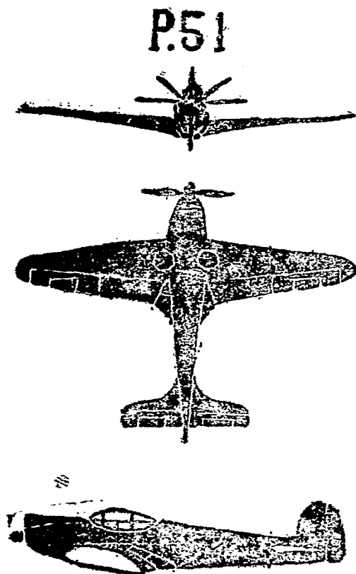
P 五十一式驅逐機（又名野馬式）（附圖一百）（三）
