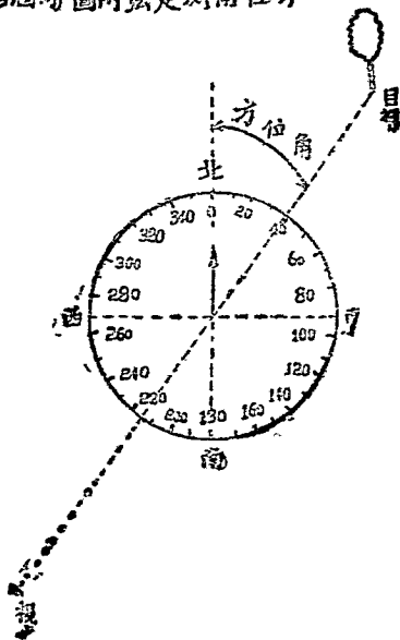
(附圖四十) 方位角测定法附圖
