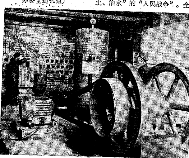
华容县地区研究材料二厂的革命职工，积极开展增产节约，不断取得新成绩。这是工人们利用废煤气机改成的空气压缩机，实现了压砖半自动化。本报记者、本报记者摄
