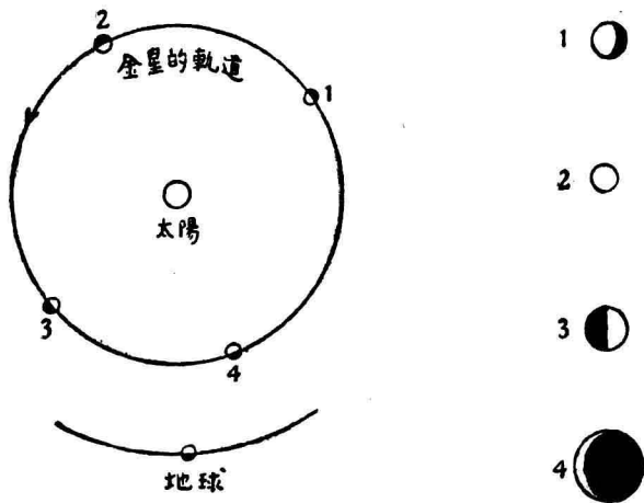
圖 一 六 金 星 的 位 相
