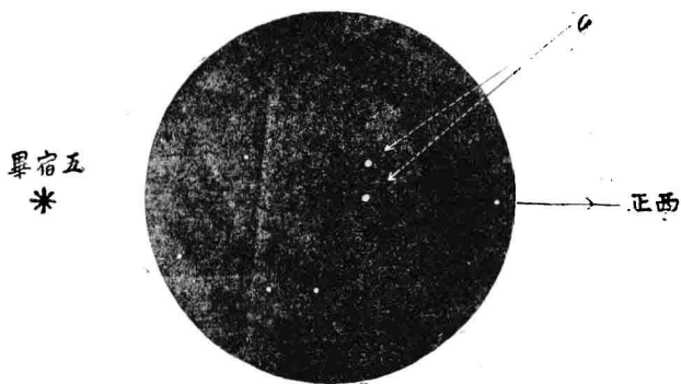
圖一八 口徑一又四分之一吋遠鏡中所見金牛座之 \theta
