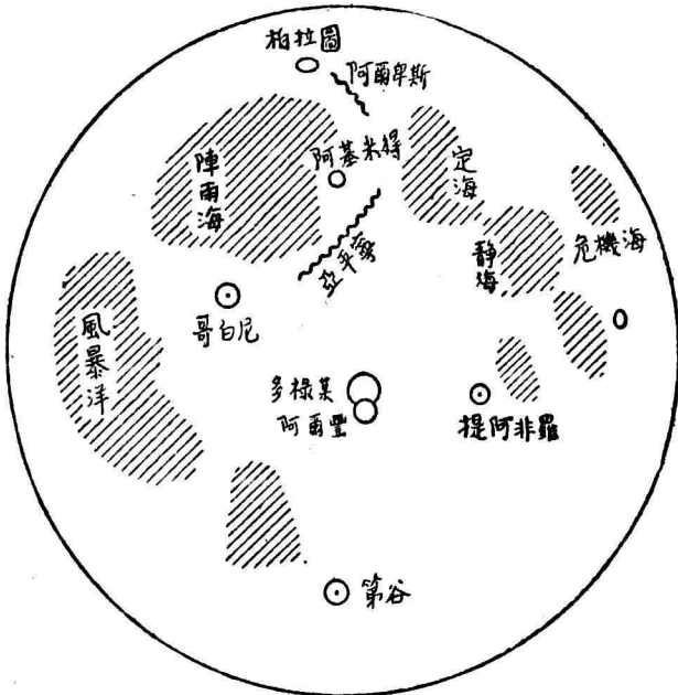
圖 一 四 月 面 圖
