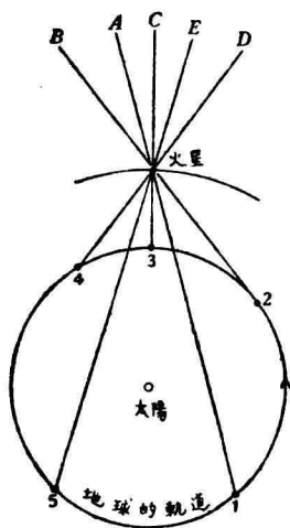
圖一二 火星的行動
