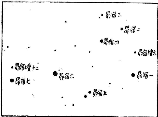
圖 一 七 昴 星 圖
