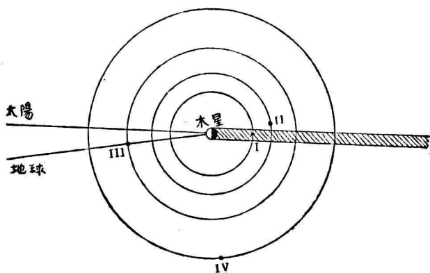
圖一五 木星的衛星 I, 蝕; II, 被掩; III, 凌犯; IV, 可見
