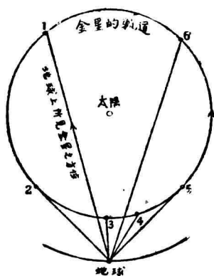
圖 一 一 金星 的 行 動
