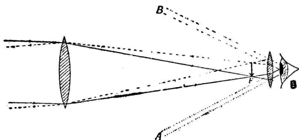
圖 一 三 天 文 遠 鏡
