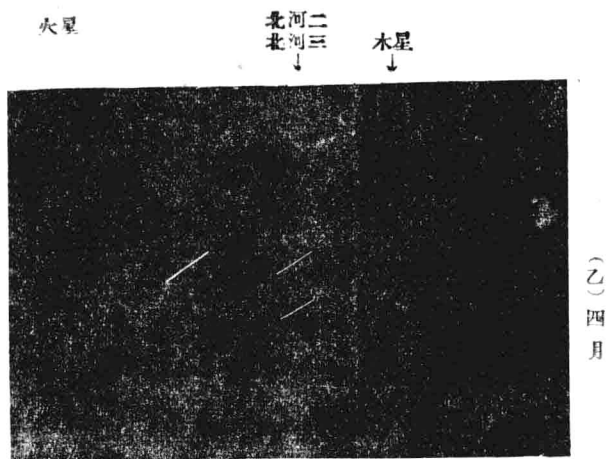
圖二一 行星的運動 (1931)
