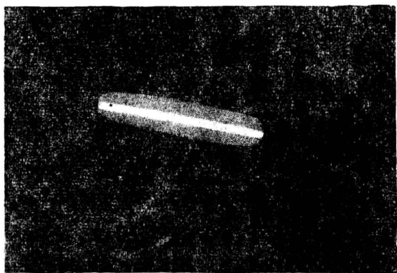
圖一九 月球行過的路線
