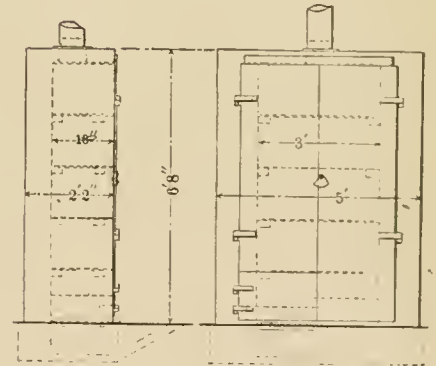
Fig. 4.—Core Oven.
