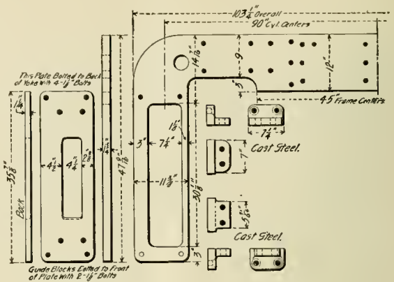
Guide Yoke.
