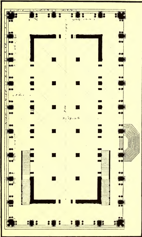
2. THE BASILICA (PALAZZO DELLA RAGIONE), VICENZA.
