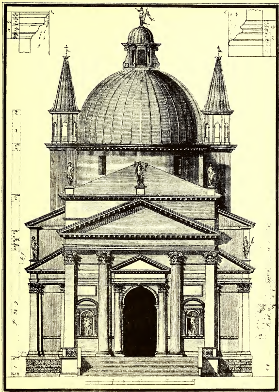
34. IL REDENTORE, VENICE.
