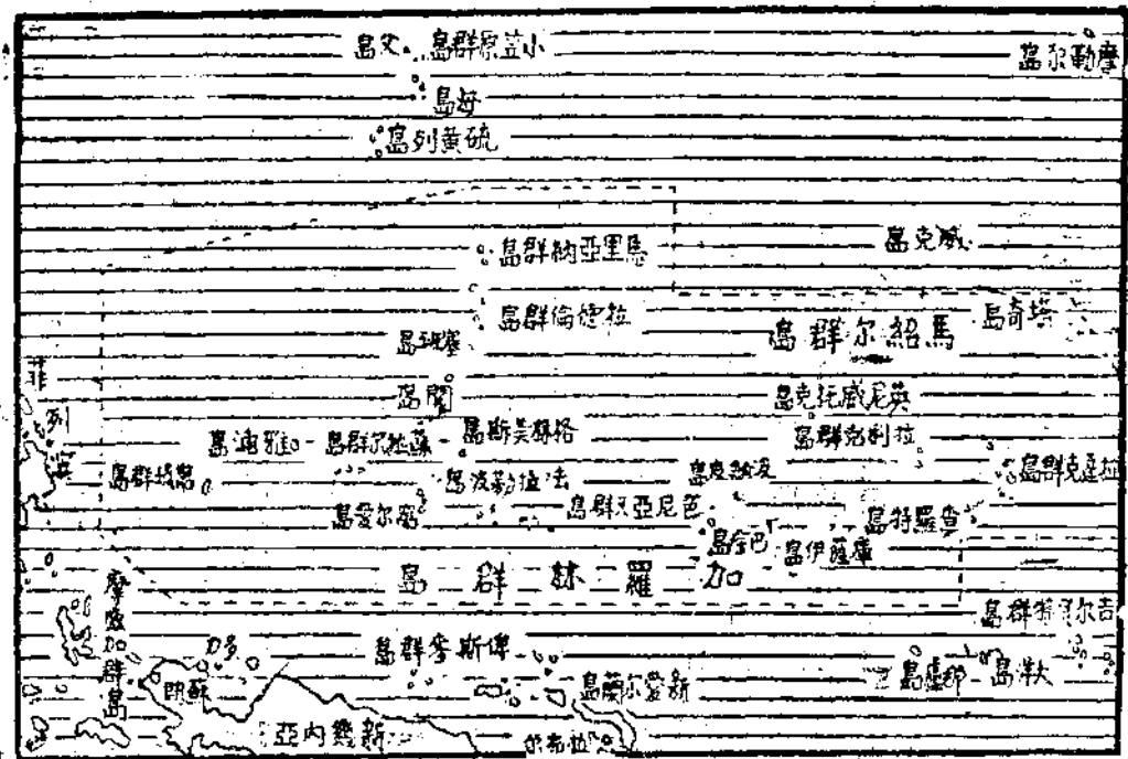
中太平洋形勢圖
