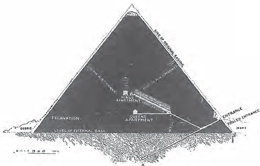
埃及基士最大金字塔的縱截面圖 第三十六圖
