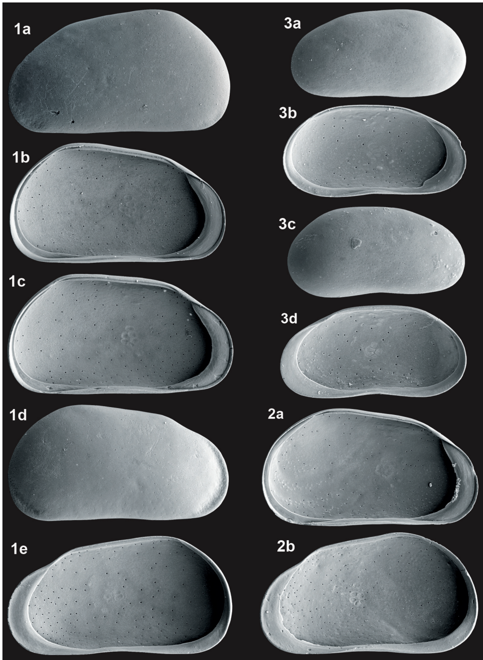
Pseudocandona sucki (HARTWIG, 1901) – Neumark-Nord (40) mWaKz Weibchen: 1a - LVa (L 0,90), 1b - LVi (L 0,90), 1c - LVi (L 0,91), 1d - RVa (L 0,90), 1e - RVi (L 0,88), Männchen: 2a - LVi (L 0,88), 2b - RVi (L 0,97).
