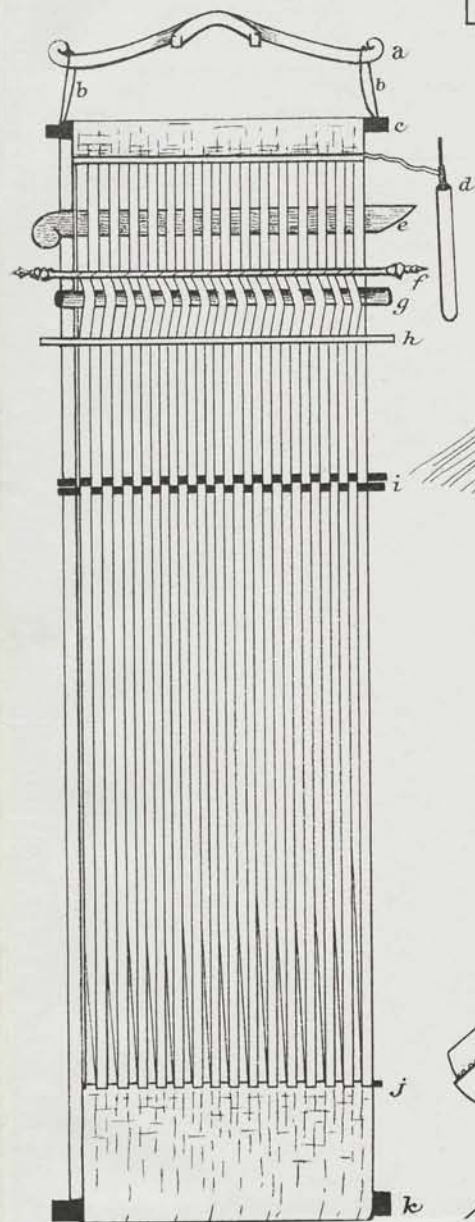
Kettingboom met losse tongen.
