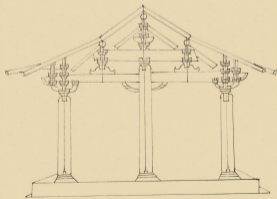
四架椽屋分心用三柱
