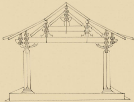
四架椽屋通檐用二柱
