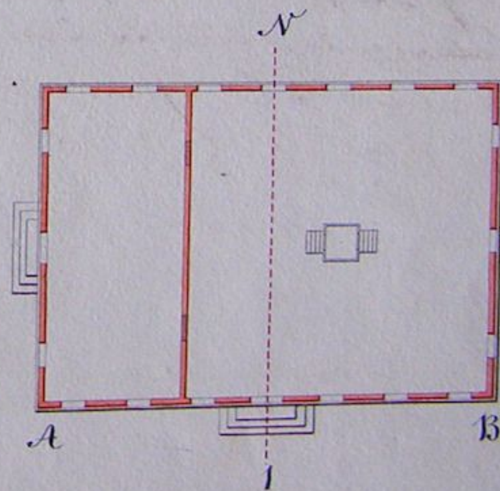
Маасштабъ къ разрѣзу и плану
