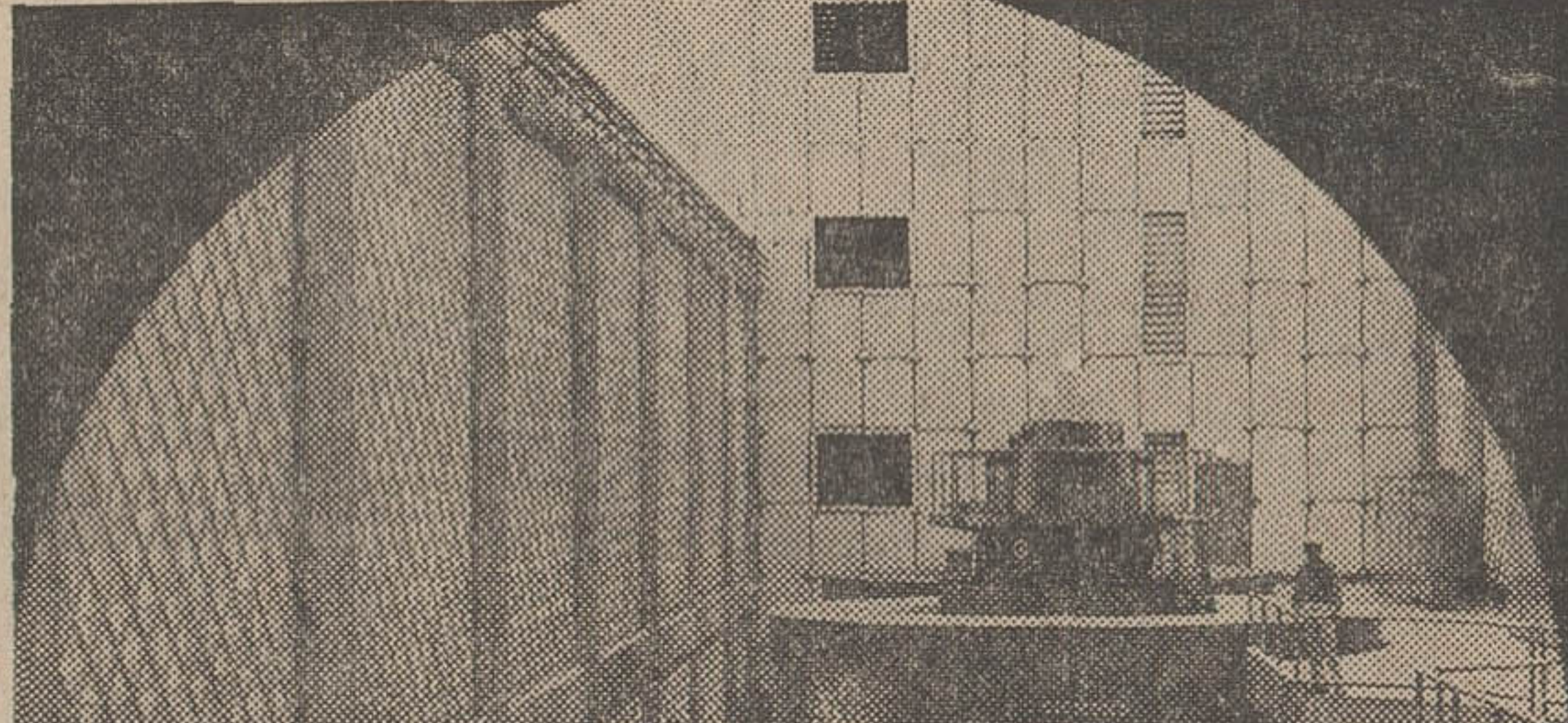
گوشه‌ای از تاسیسات سد عظیم محمد رضا شاه پهلوی در این عکس دو دستگاه از چهار دستگاه مولد برق ۶۶۰ کیلوواتی زیمنس دیده میشود .
