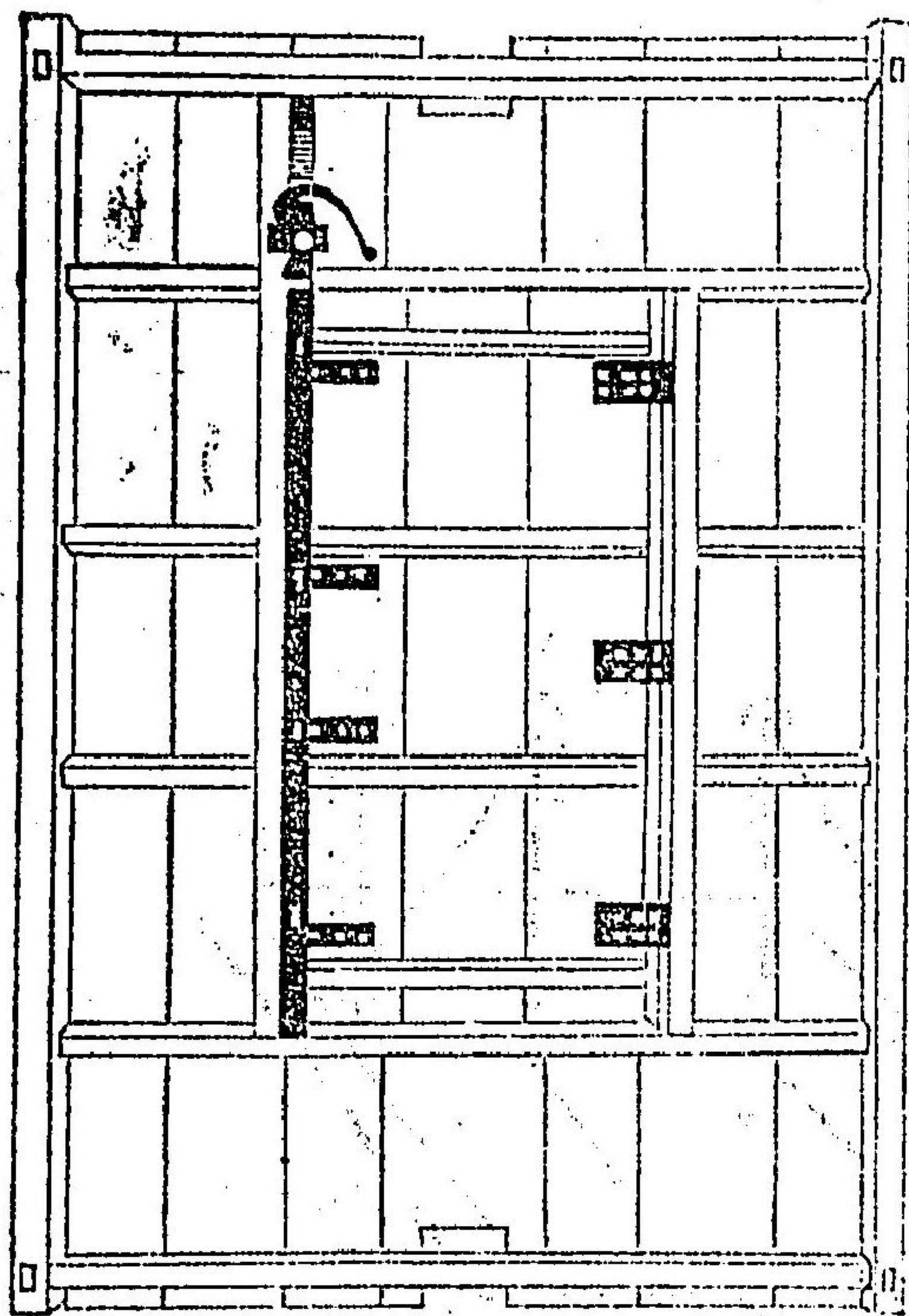
機車裝置圖實物 三十分ノ一
