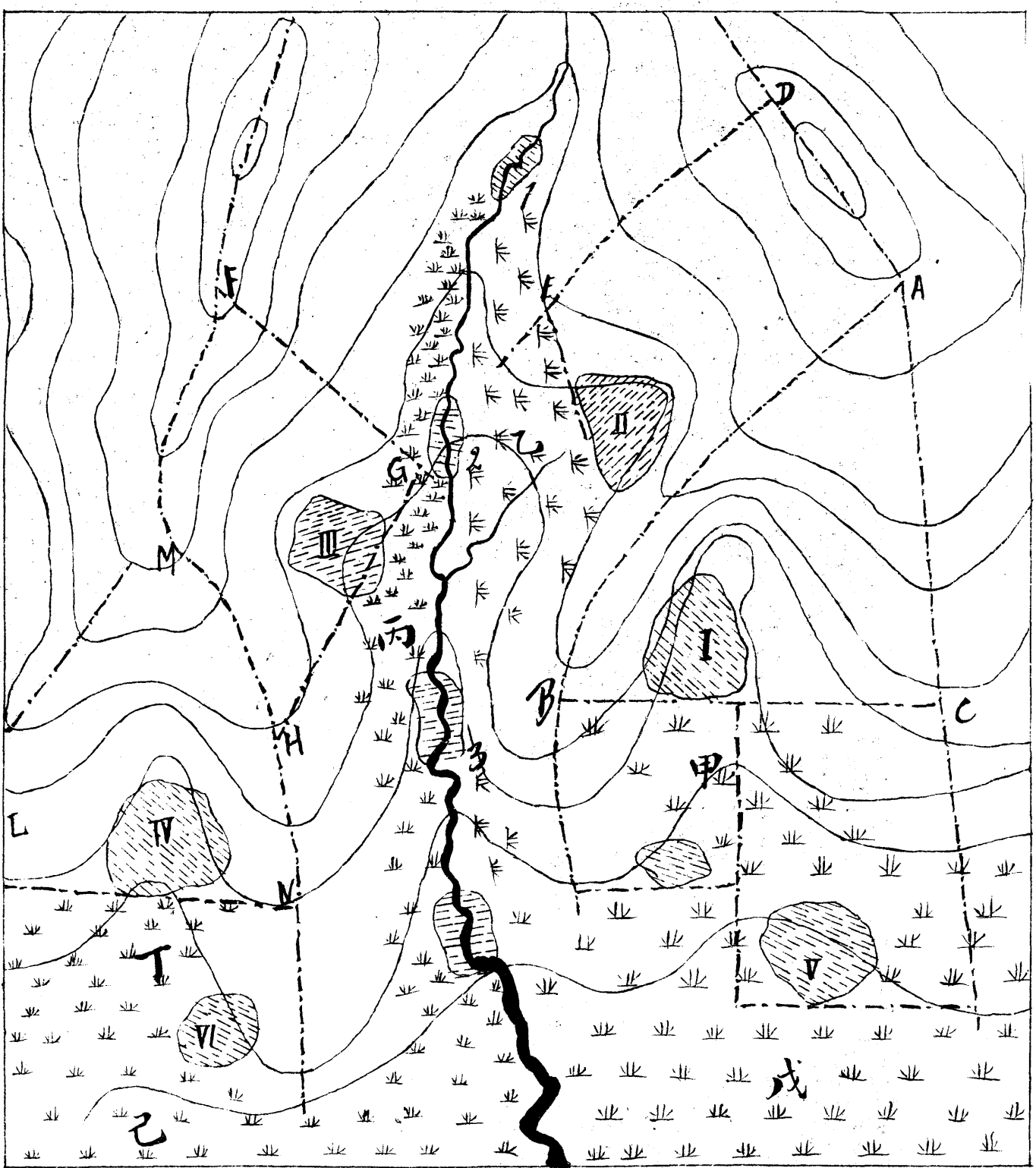
(圖一第)圖配分之壩堰塘
