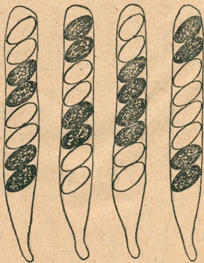
第十三圖 Neurospora sitophila 之子囊內二種異性孢子之排列(模 擬圖)。
