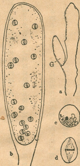
第七圖 水松(Codium tomentosum)之大接合子囊之發生： a 外形，G 為大接合子囊； b 大接合子囊之縱斷面（核正演異型分裂）； c 凝聚時期； d 異型核分裂中期。（威廉氏千九百二十五年）
