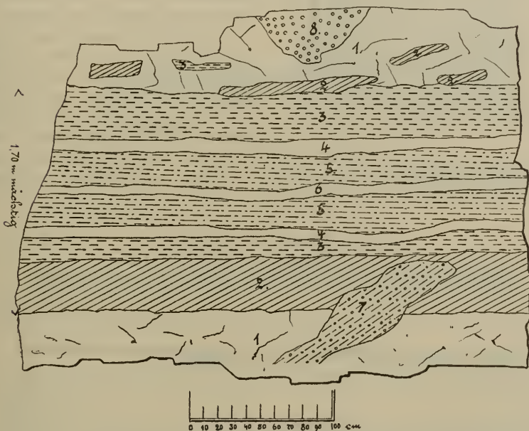
Fig. VIII. Erster Hangendschlag auf dem Rudolf-Horizont. Ortsstoss, Hangendgang.
