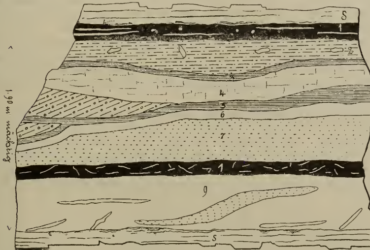
Fig. XI. Abbauort Nr. 7 auf dem Rudolf-Horizont. Ortsstoss, Hangendgang (Anfang August 1890), 1:20.
