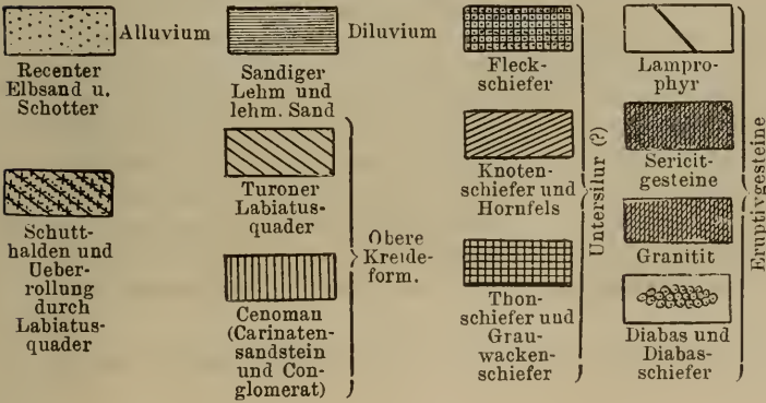
Geologische Karte des Elbthales nördlich von Tetschen. Maassstab 1 : 33.000.
