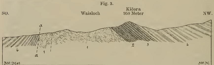
Durchschnitt der Rauschenbacher Insel, westlich vom Zeleznybache, in der Gegend Waisloch und Kičora. Maassstab 1 : 25000.
