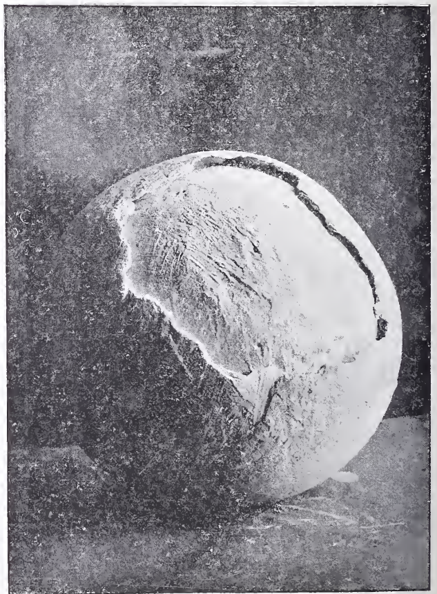
FIGURE 2. — Imitation expérimentale de l'orogénie de l'Europe.
