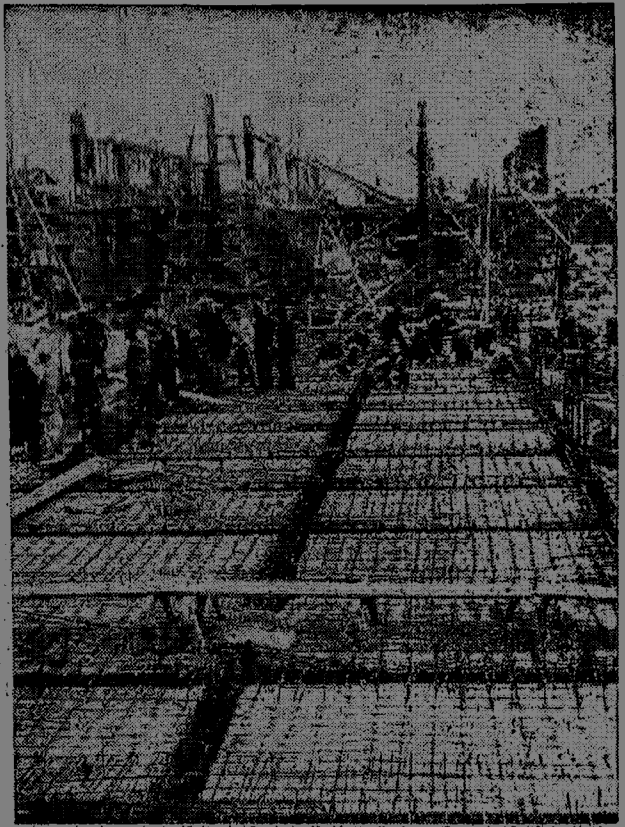
建立在湘潭河東區的湘潭棉紡織廠，是一座規模宏大的現代化棉紡織廠，由於今年部分開工生產，現在工程正進入緊張的階段。這是正在進行中的該廠基礎開工的情形。
