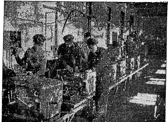
張大機十八廠制工車開制善小組學習先進經驗，創造流水作業法。這種工作方法是將工作物放在裝有四個小輪的木板上，下面鋪有軌道，一道工序完畢後，只要用手一推，就把工作物送給下一道工序。這樣，可使生產效率提高兩倍。
