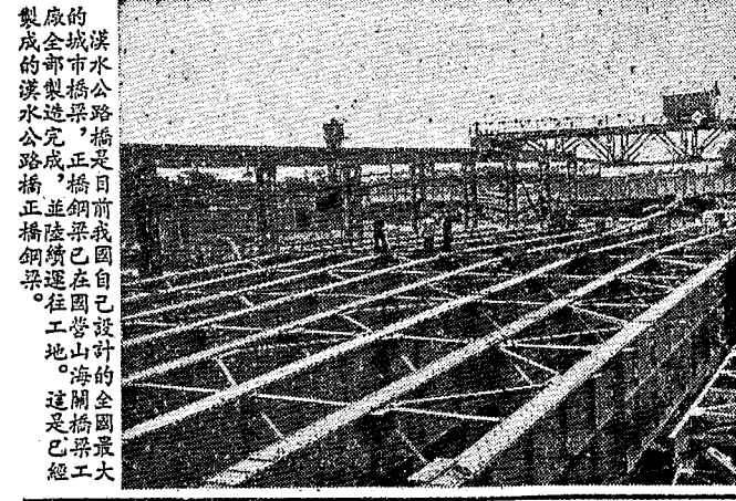
漢水公路橋樑工程我國自己設計的全國最大規模的橋樑工程。在國營湖南鋼鐵廠生產的橋樑鋼材，已運到現場。
