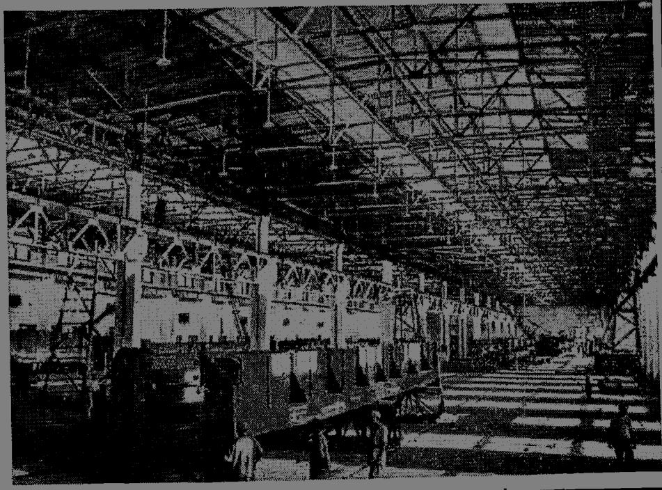
△ 去年五月開始建設的華北金屬結構廠，廠房工程已經完工，工人正在安裝機器。這個廠是根據蘇聯最新標準設計進行建設的。它投入生產後，將大量生產鋼房架、鋼柱、工業管等，供應華北各地工業建設需要。 新華社記者喻忠如攝
