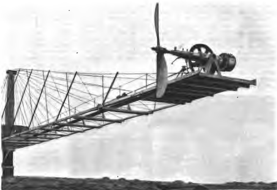
Снарядъ для испытанія воздушныхъ винтовъ.
