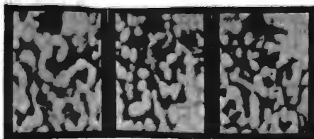
Рис. 2. Грануляція солнечной поверхности, по А. П. Ганскому.
