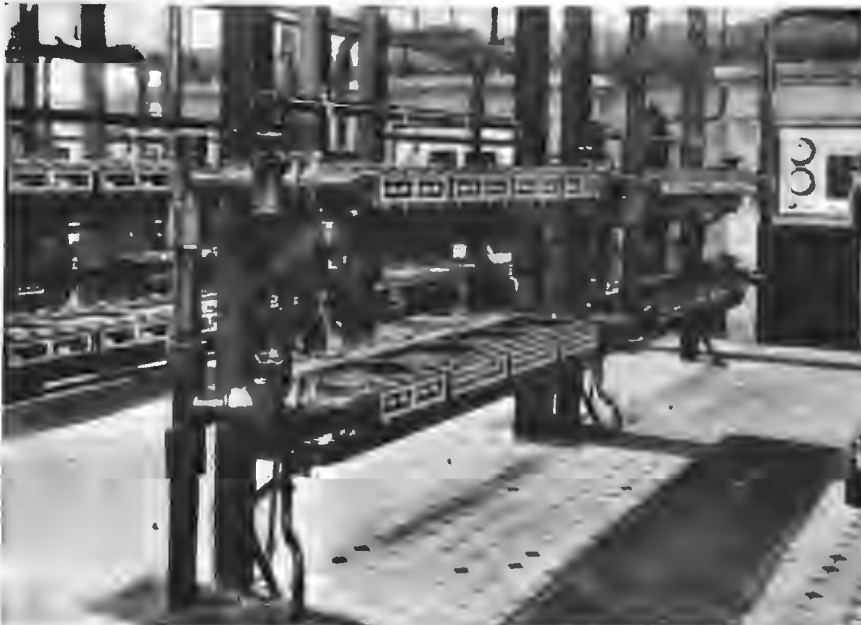
Аппараты, посредствомъ которыхъ проточная вода озонируется подѣ дѣйствіемъ сильныхъ электрическихъ токовъ.
