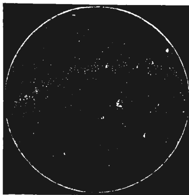
Рис. 2. Общій видъ Млечнаго пути къ Южному полушарію.
