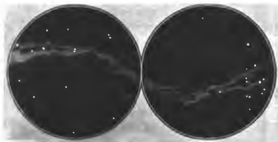
Место появления новых звезд на небе.
