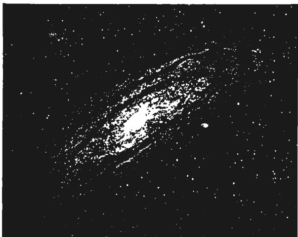
Рис. 1. Туманность въ Андромедѣ.
