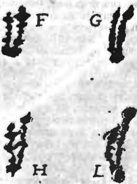
Рис. 1. Первые рисунки солнечныхъ пятенъ Галилея.
