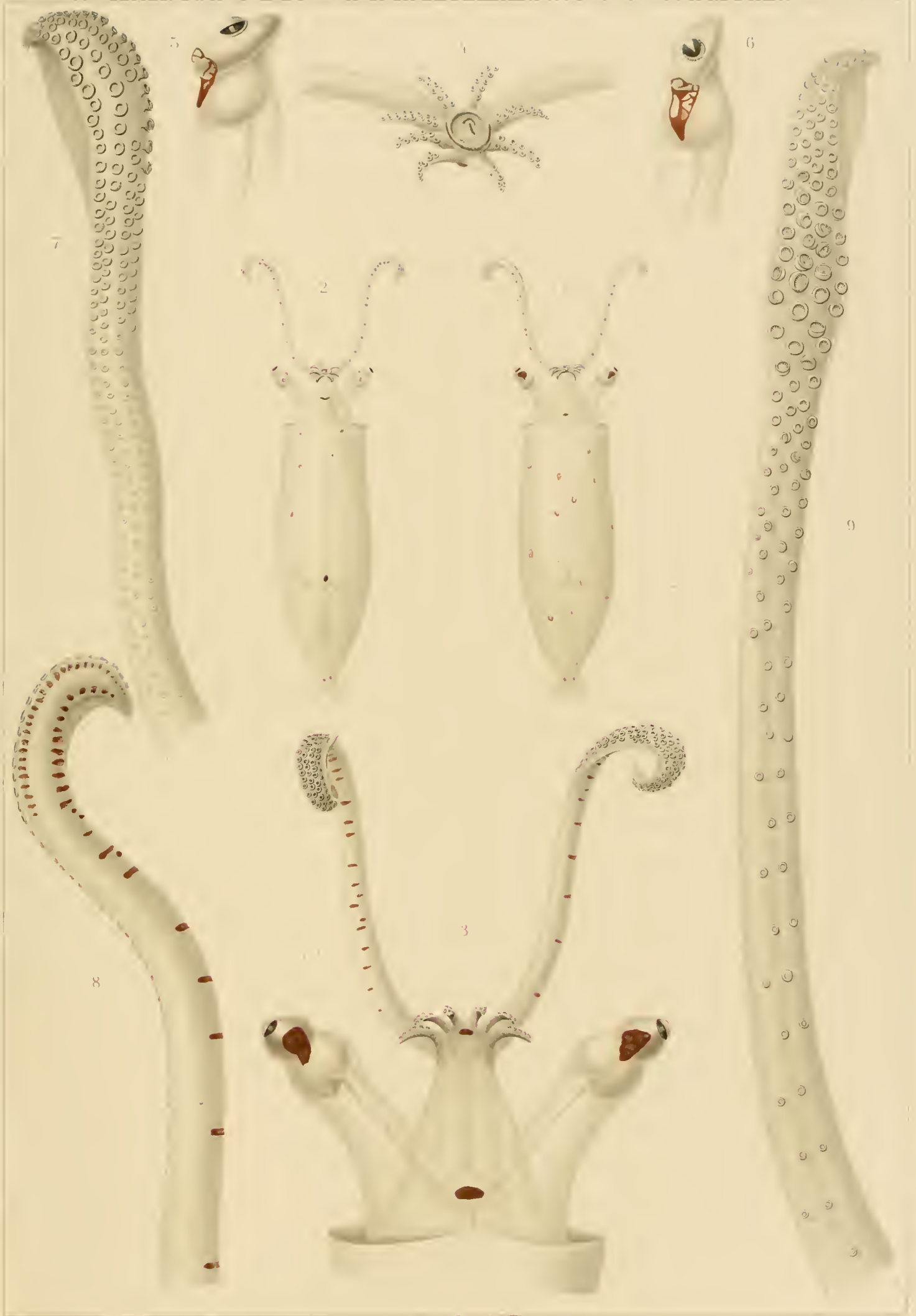
lat. 1. Corynomma speculatum
