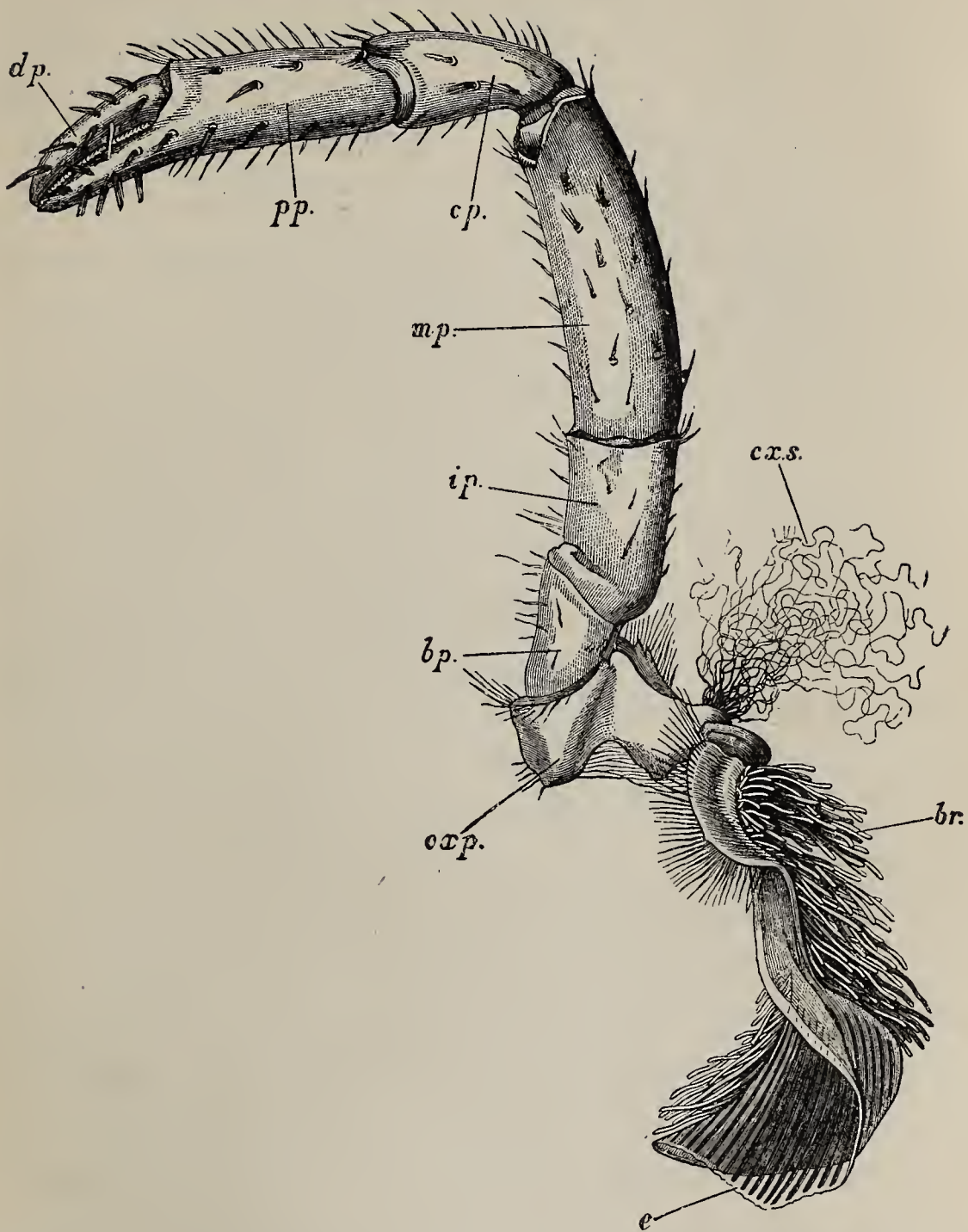
FIG. 46.— Astacus fluviatilis .—The second ambulatory leg of the left side ( \times 3 ). cxp , coxopodite ; bp , basipodite ; br , gill ; cx.s. , coxo-poditic setæ ; e , lamina of gill or epipodite ; ip , ischiopodite ; mp , meropodite ; cp , carpopodite ; pp , propodite ; dp , dactylopodite.
