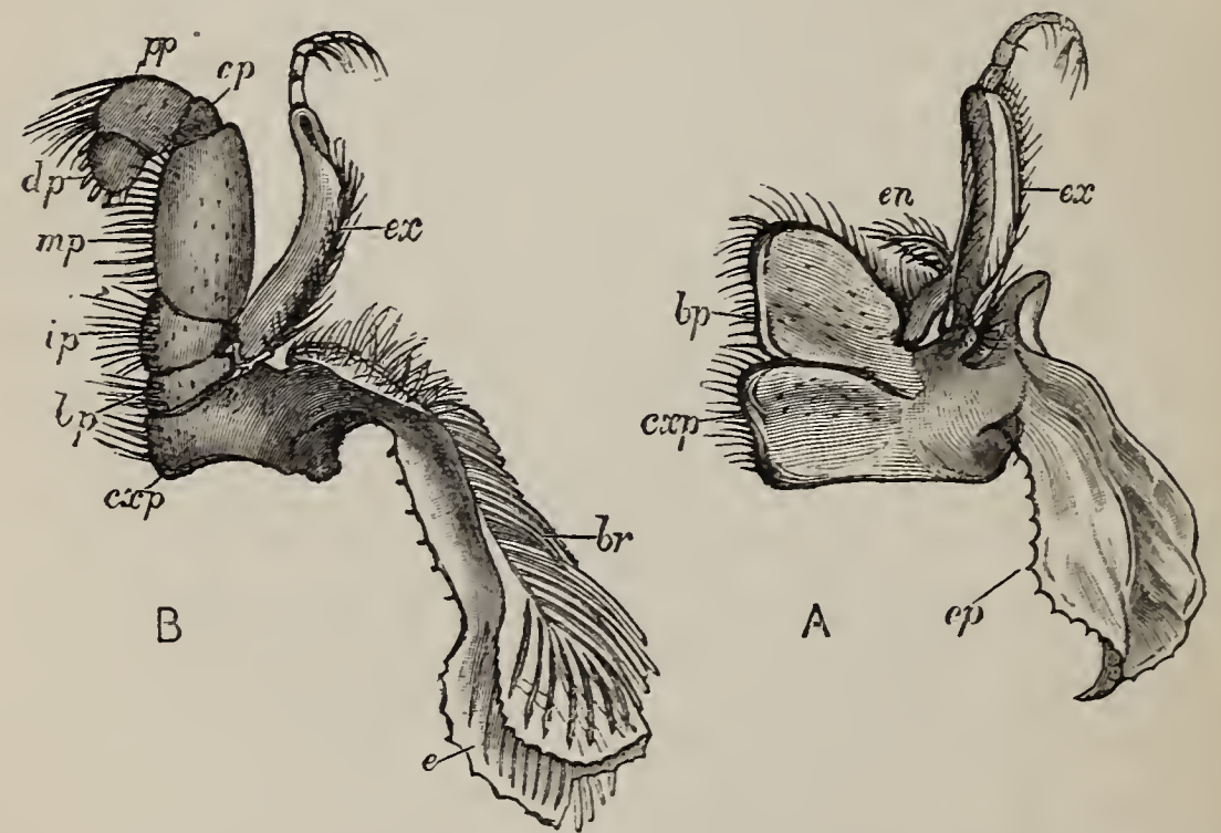
FIG. 45.— Astacus fluviatilis .—A, the first; B, the second maxillipede of the left side ( \times 3 ). csp , coxopodite; bp , basipodite; e , br , podobranchia; ep , epipodite; en , endopodite; ex , exopodite; ip , ischiopodite; mp , meropodite; cp , carpopodite; pp , propodite; dp , dactylopodite.
