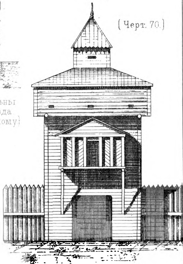
Проезжая башня въ г Илимскъ. (по Ласковскому.)
