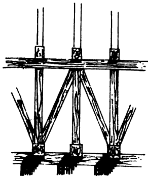
( Черт. 128 )
