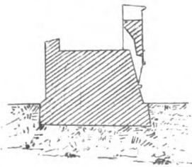
Разрѣзь стѣны Китая-города (по Ласковскому.)
