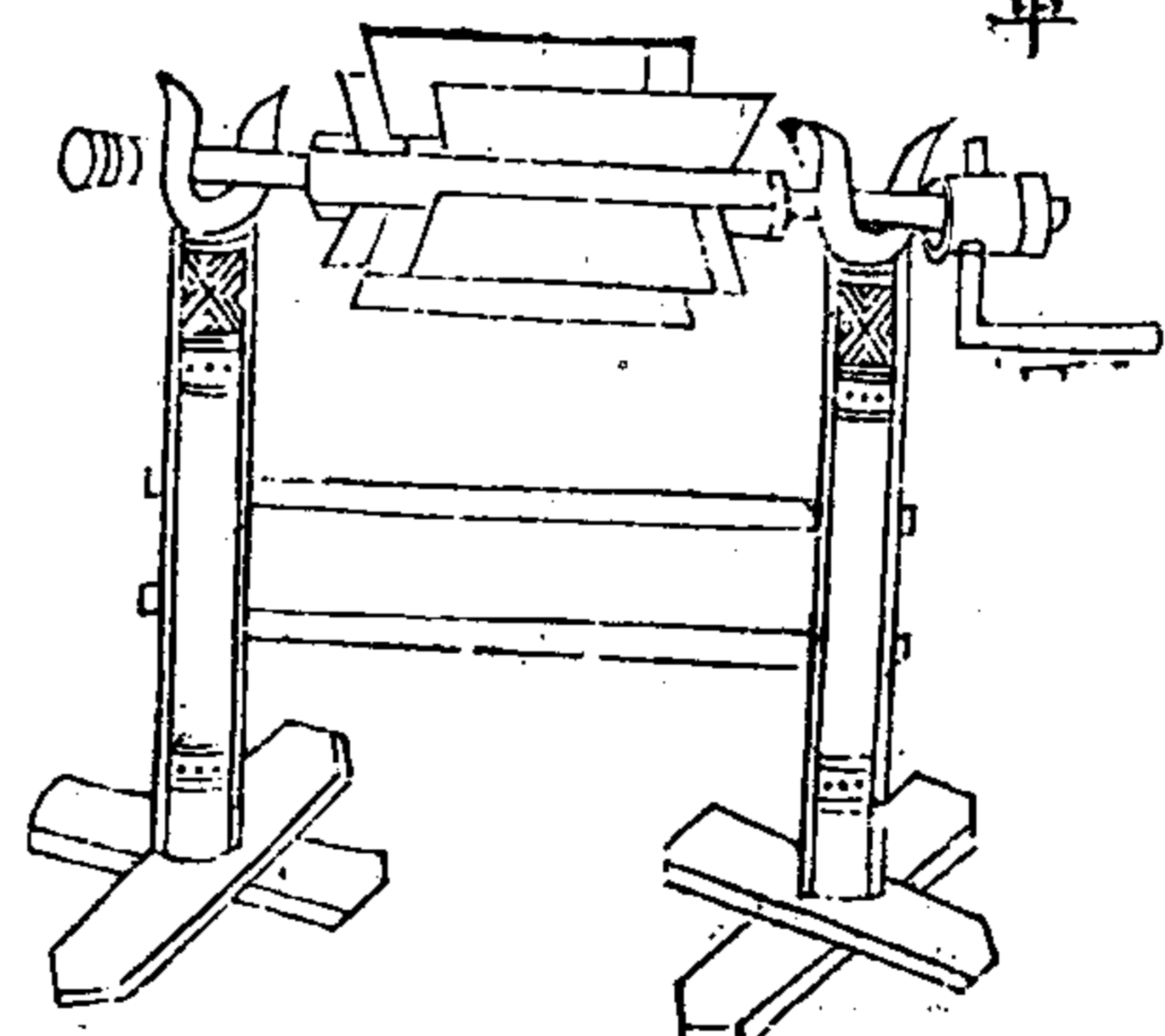
風扇車
