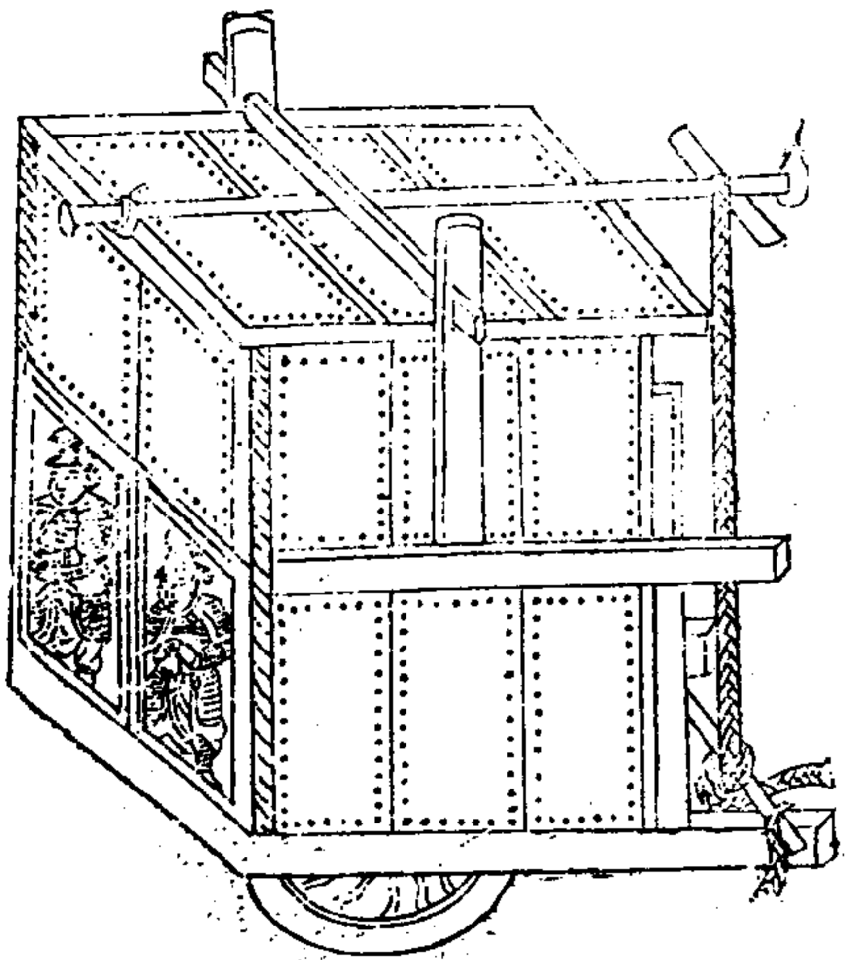
填壕皮車
