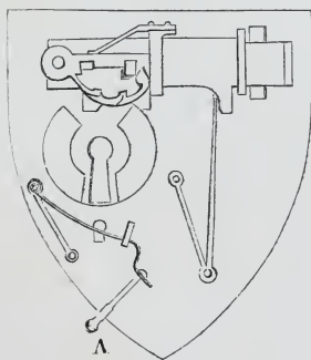
SERRURE A BOSSE. XIV e SIECLE
