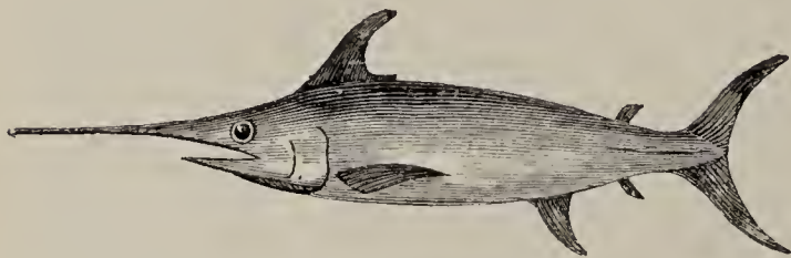
FIG. 224.—Sword-fish ( Xiphias ).
