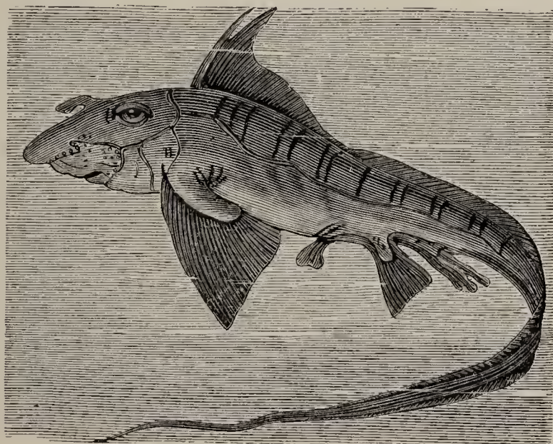
FIG. 203.—The Chimæra .
