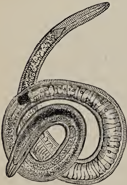
FIG. 43.— Trichina .
