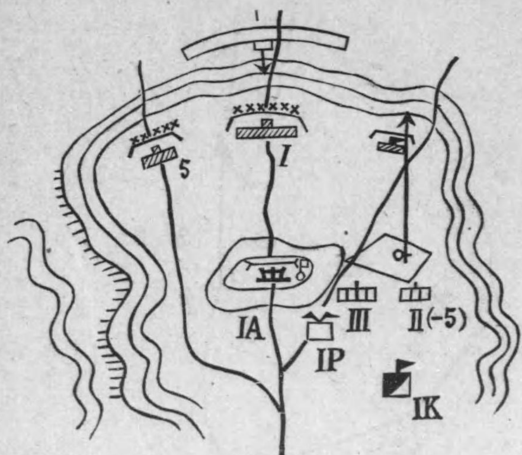
◎高地縁端ノ攻勢防禦ノ例
