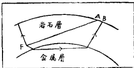
第一圖 地震行經
