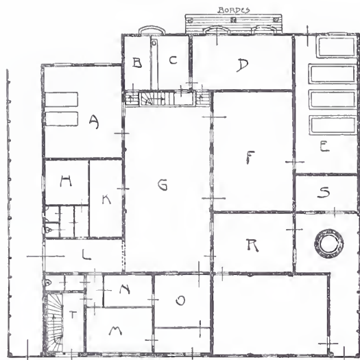
Nieuwe Melkinrichting „Arnhem”. Plan gelijkstraats. Schaal 1 à 400.
