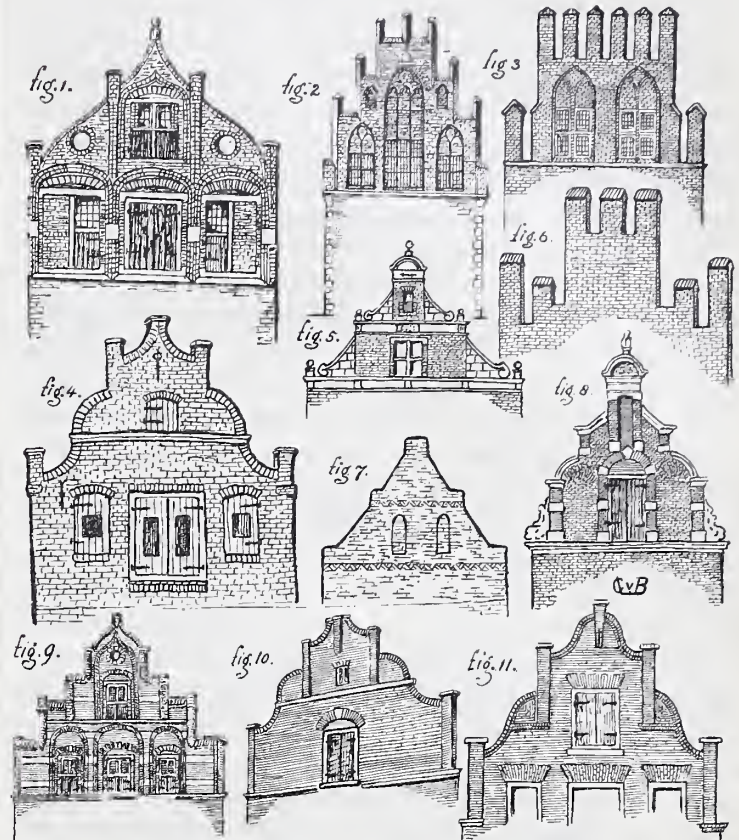
Schetsteekeningen van Gothieke en Renaissance-gevels in het Oosten van Gelderland.
