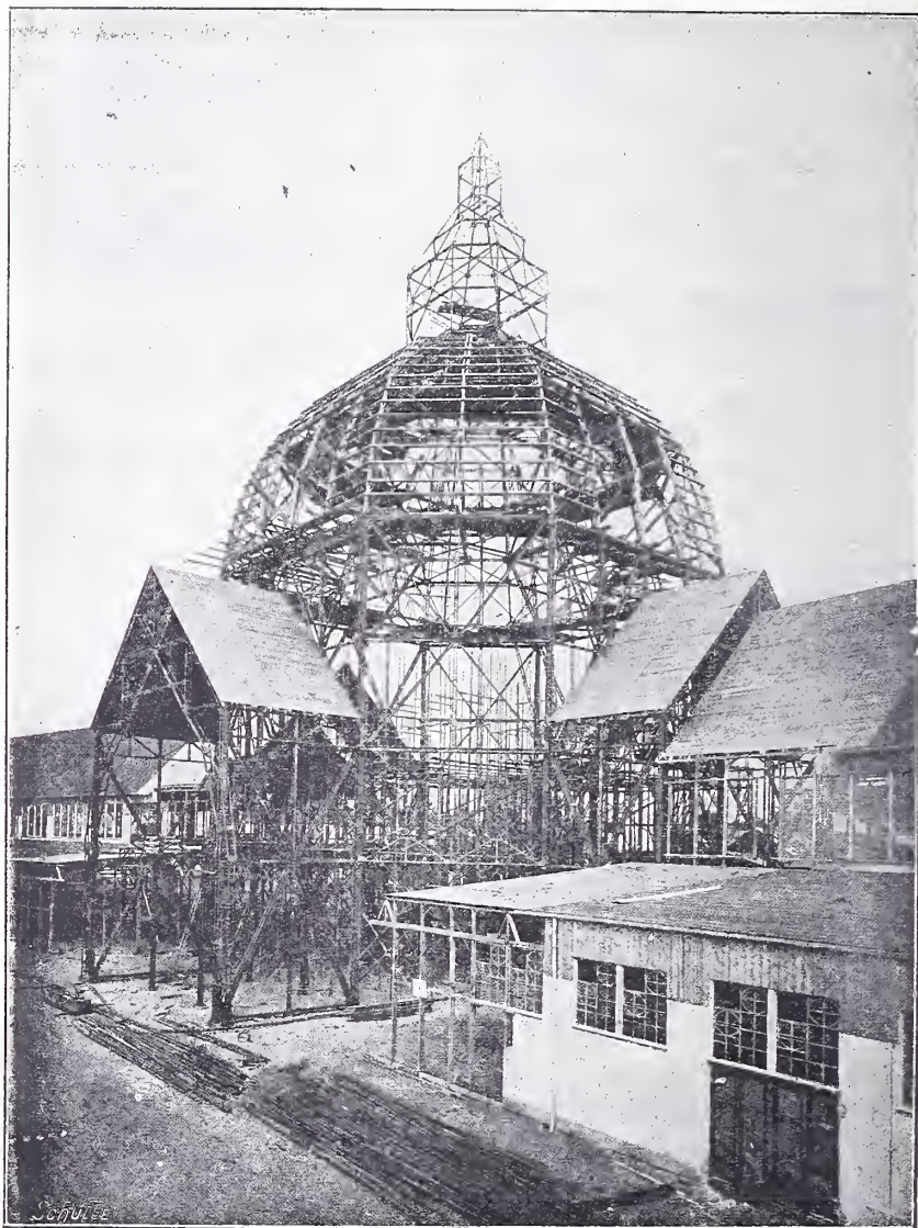
Koepel van het Hoofdgebouw der Tentoonstelling te Düsseldorf, in 1902.
