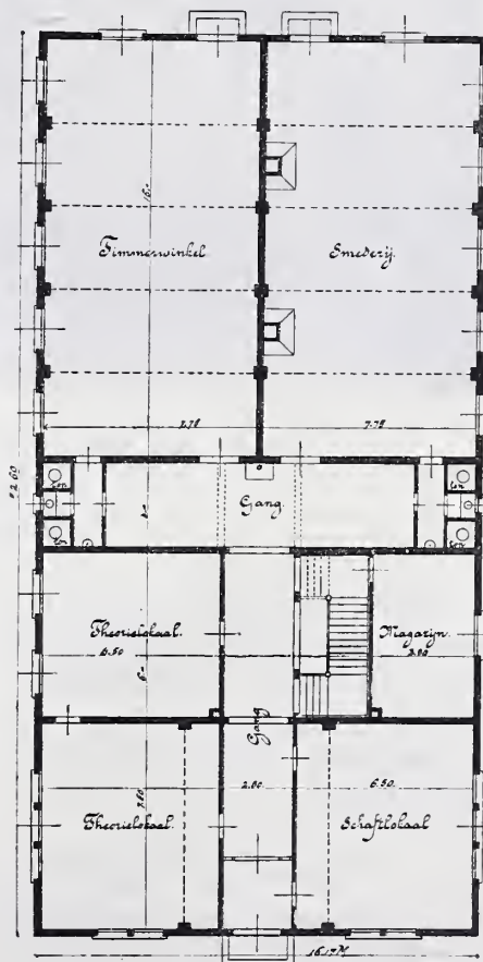
Ambachtsschool te Middelharnis. Beganegrond. Schaal 1 à 300.
