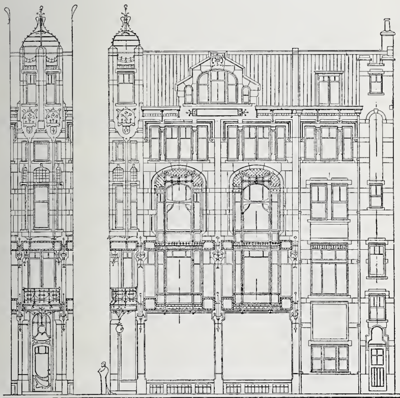
Ontwerp van den architect Joseph Herman. Schaal 1 à 200.
