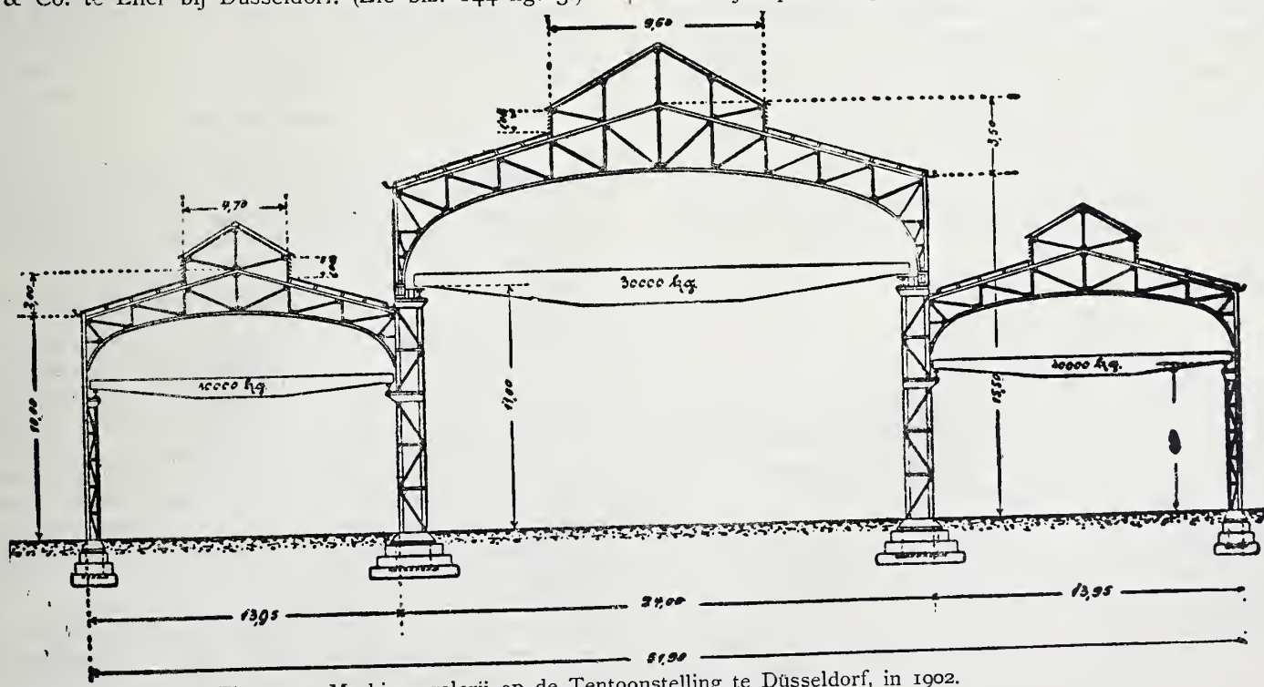
Fig. 2. Machinen-galerij op de Tentoonstelling te Düsseldorf, in 1902. Dwarsdoorsnede.
