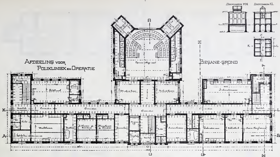
Afdeling Vroedkunde en Vrouwenziekten. Schaal 1 à 500.
