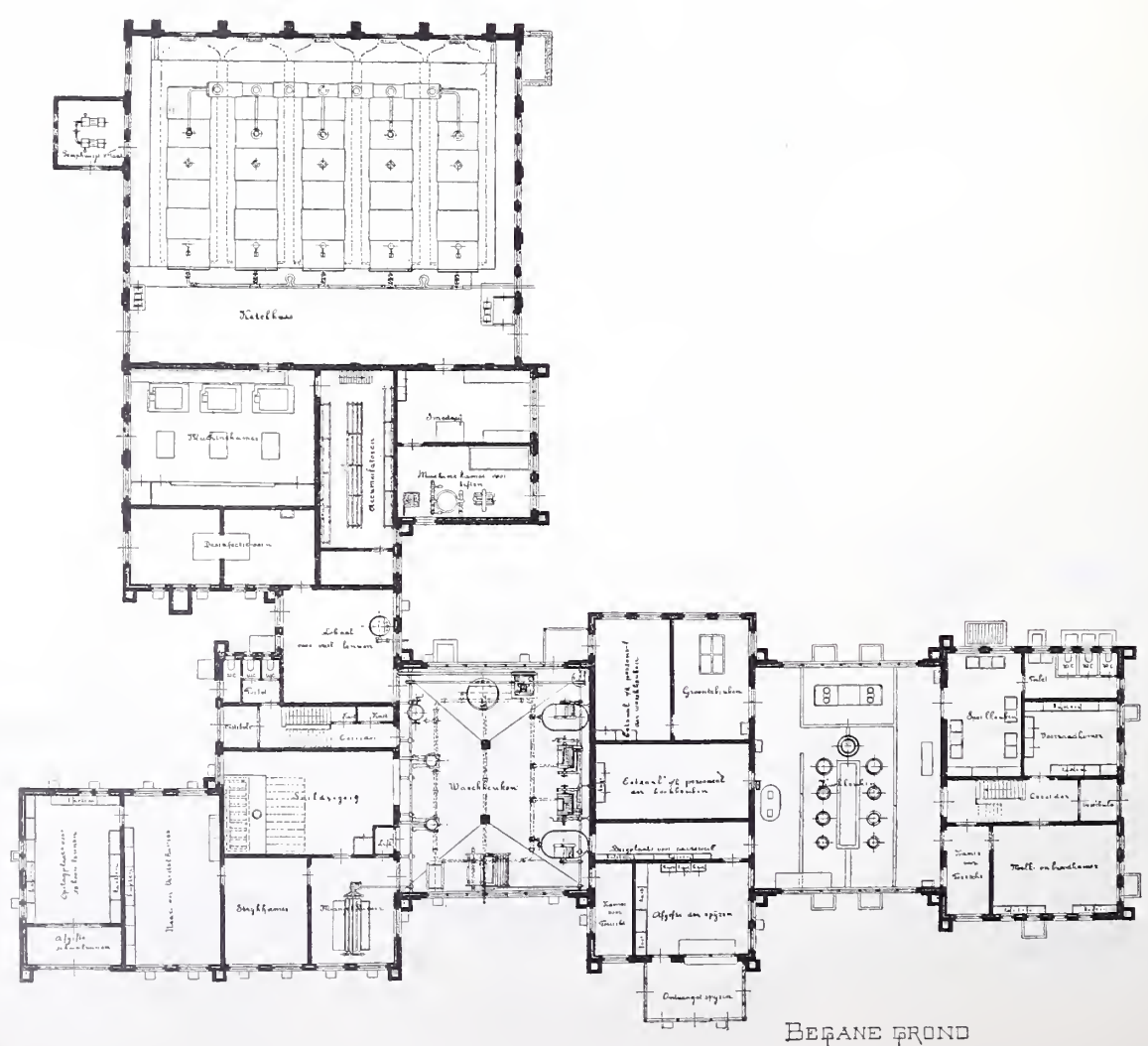
Wasch- en Kookgebouw en Ketelhuis. Schaal 1 à 400.
