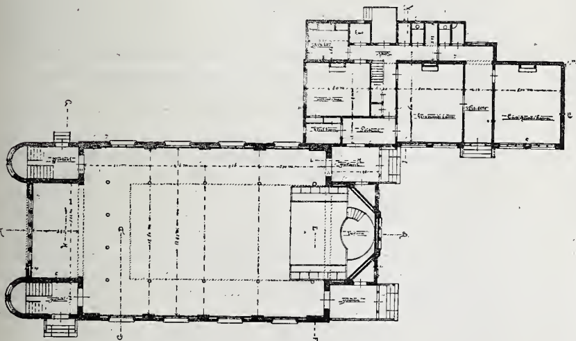
Plattegrond, ontwerp, motto: Salomo 24 vs. 3. Schaal 1 à 400.
