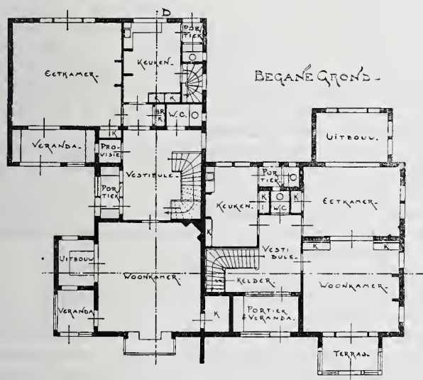
Dubbele Villa te Laren N. H. Schaal 1 à 300.
