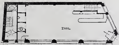
Indeeling v. d. Beganegrond. Schaal 1 à 300.
