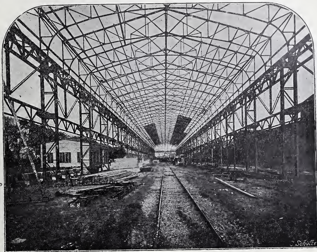
Fig. 1. Binnenaanzicht van de Machinen-galerij op de Tentoonstelling te Düsseldorf, in 1902.
