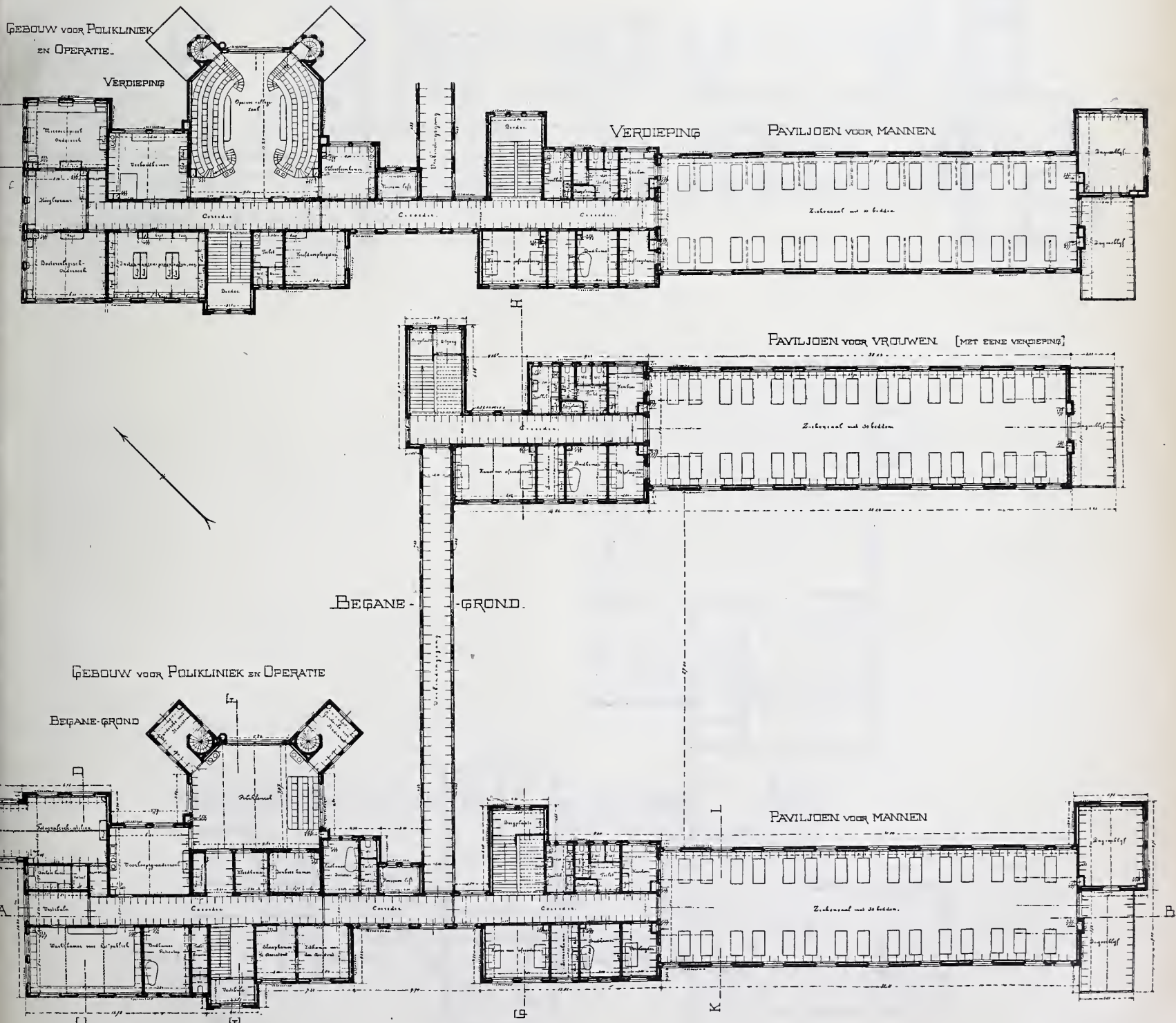
Chirurgische Afdeling. Schaal 1 à 400.
