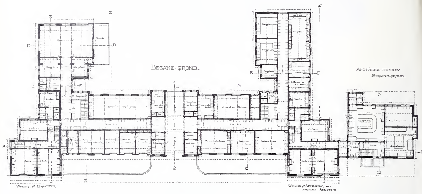
Administratiegebouw. Schaal 1 à 400.
