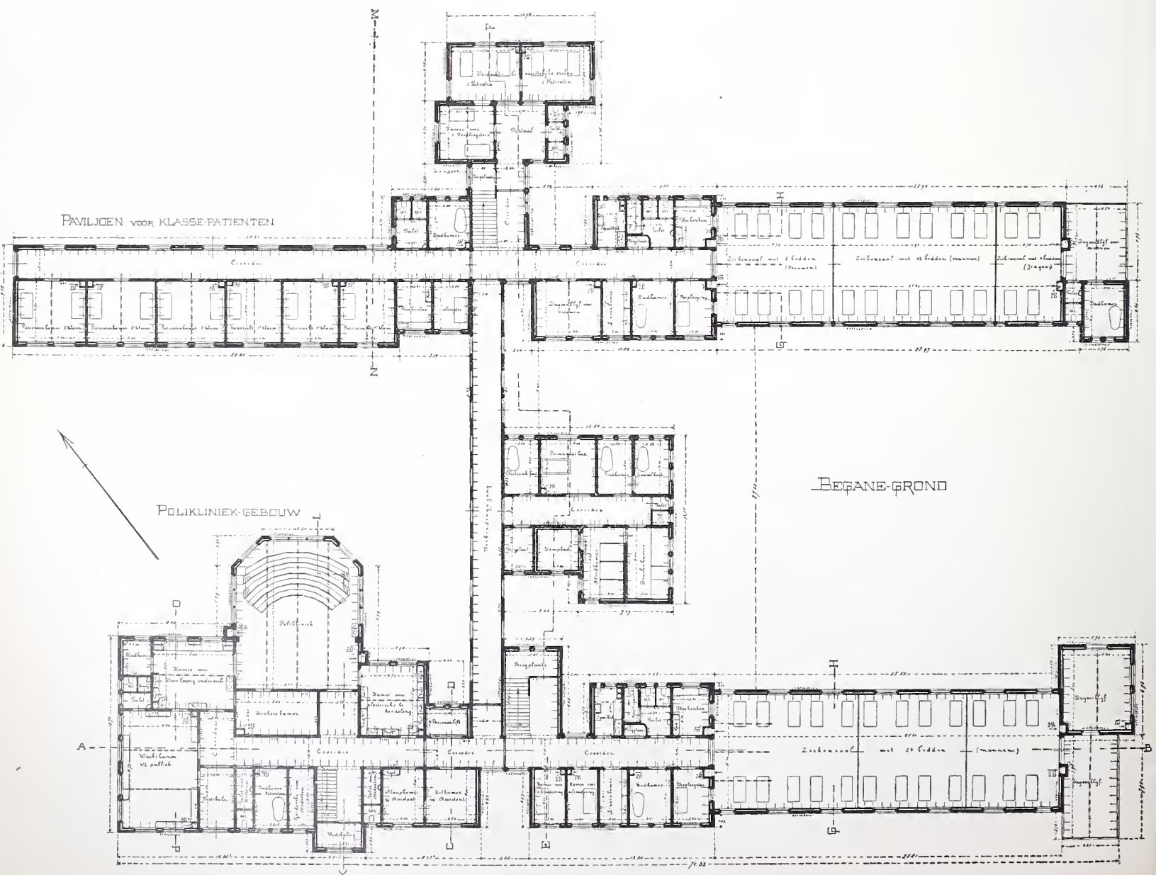
Medische Afdeling. Schaal 1 à 400.
