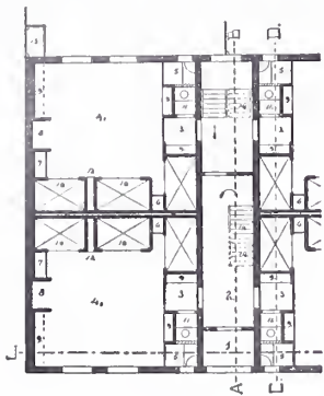
Plan beganegrond. Schaal 1 à 300.
