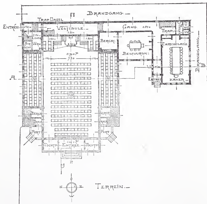
Plattegrond, ontwerp, motto: Centraalbouw. Schaal 1 à 400.
