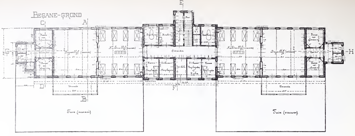
Psychiatrische Afdeeling. Schaal 1 à 400.
