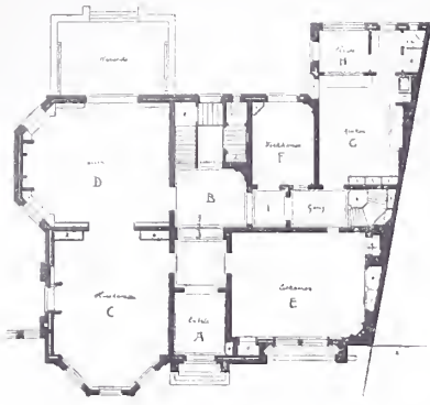
Villa aan de Paviljoenslaan te Haarlem.
