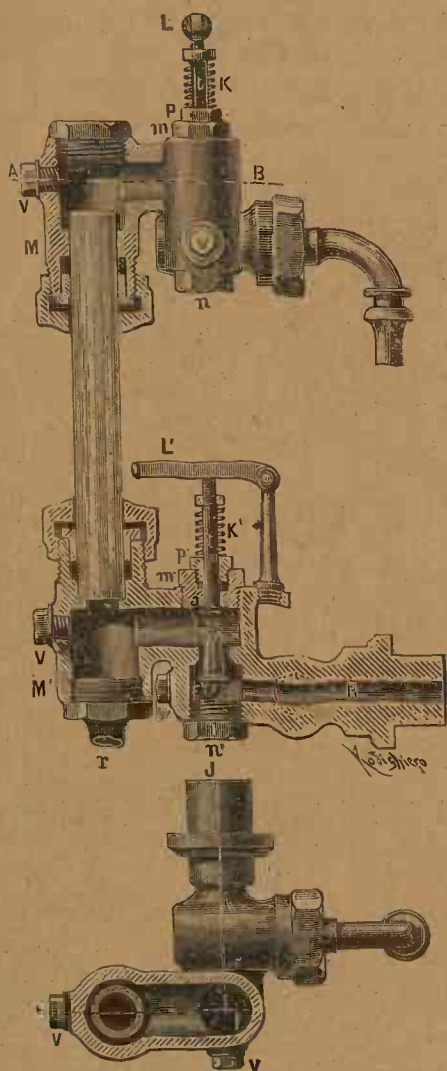
Nivelul de apă cu supapa automată.
