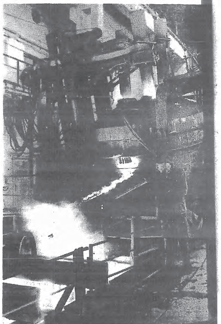
南烏拉爾的煉鎳聯合廠。 這是電爐煉鎳的工場間， 鎳液正由爐中傾出。
