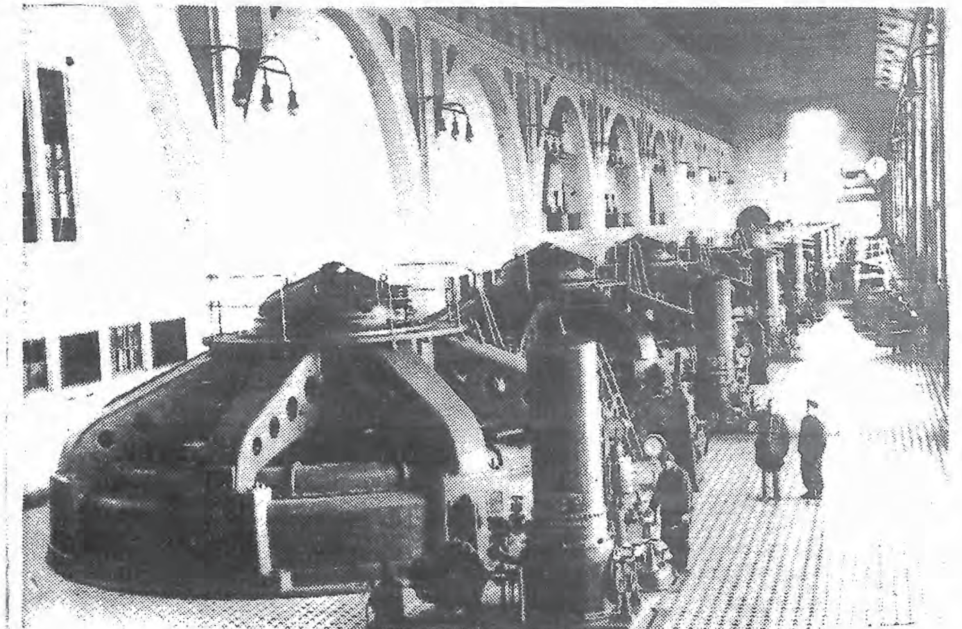
伏耳霍夫列寧水力發電廠 的機器房。
