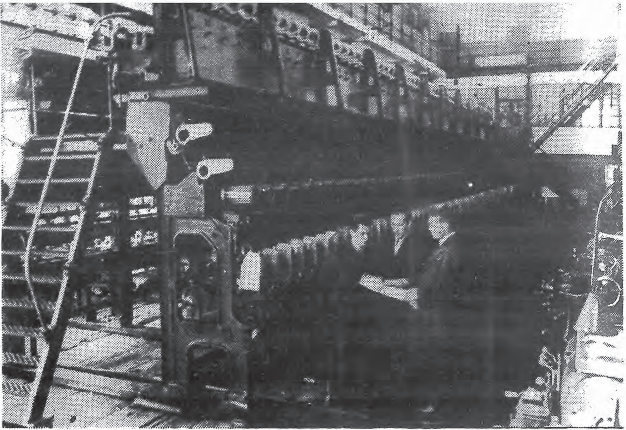
莫斯科紡織機器實驗工廠的新式紡織聯合機。該機把六種動作合在一起，專紡人造絲。這是在裝運前的最後檢查。
