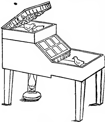
BROODER.—FIG. 4.
