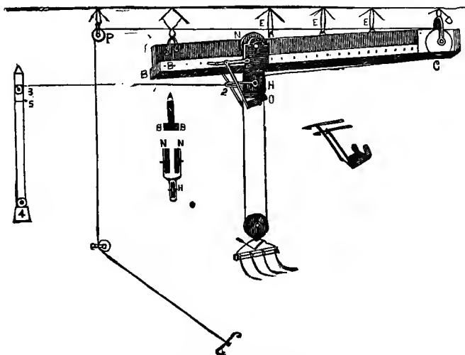
HAY ELEVATING APPARATUS.
