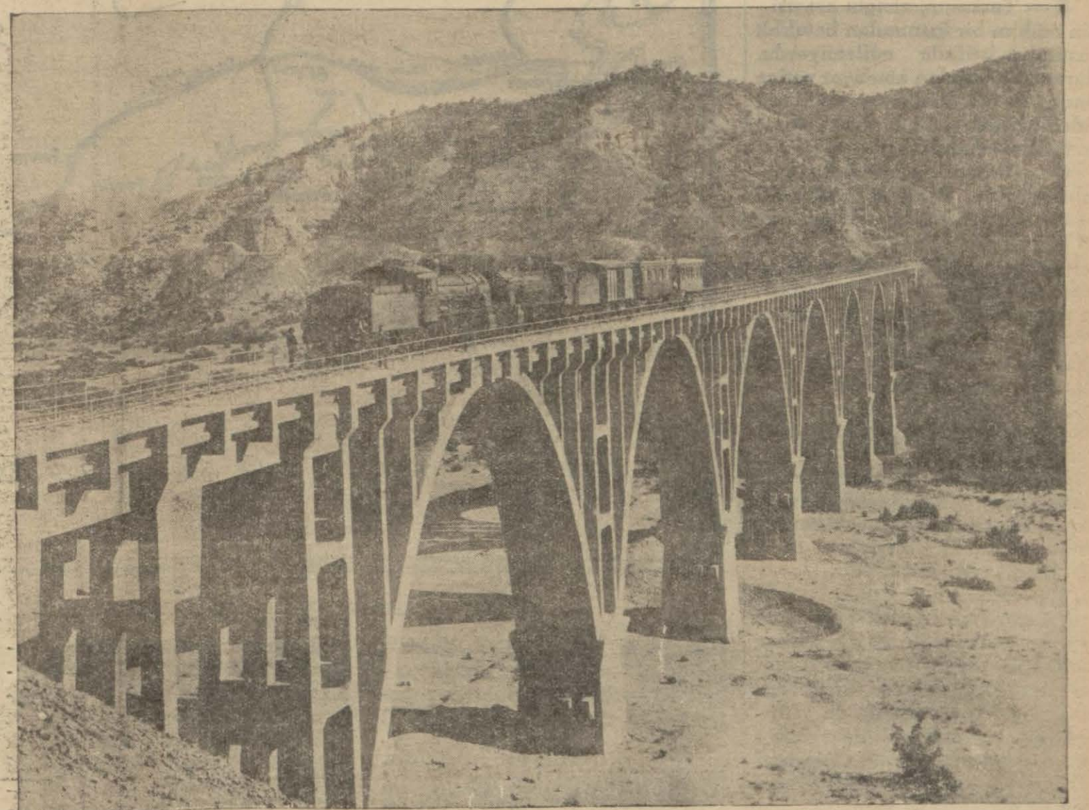
Fevziyapaşa - Diyarbakir hattında Türkiyenin en büyük şimendifer köprüsü. Bu köprüünün 300 metre uzunluğa ve 30 metre yüksekliğe vardır.
