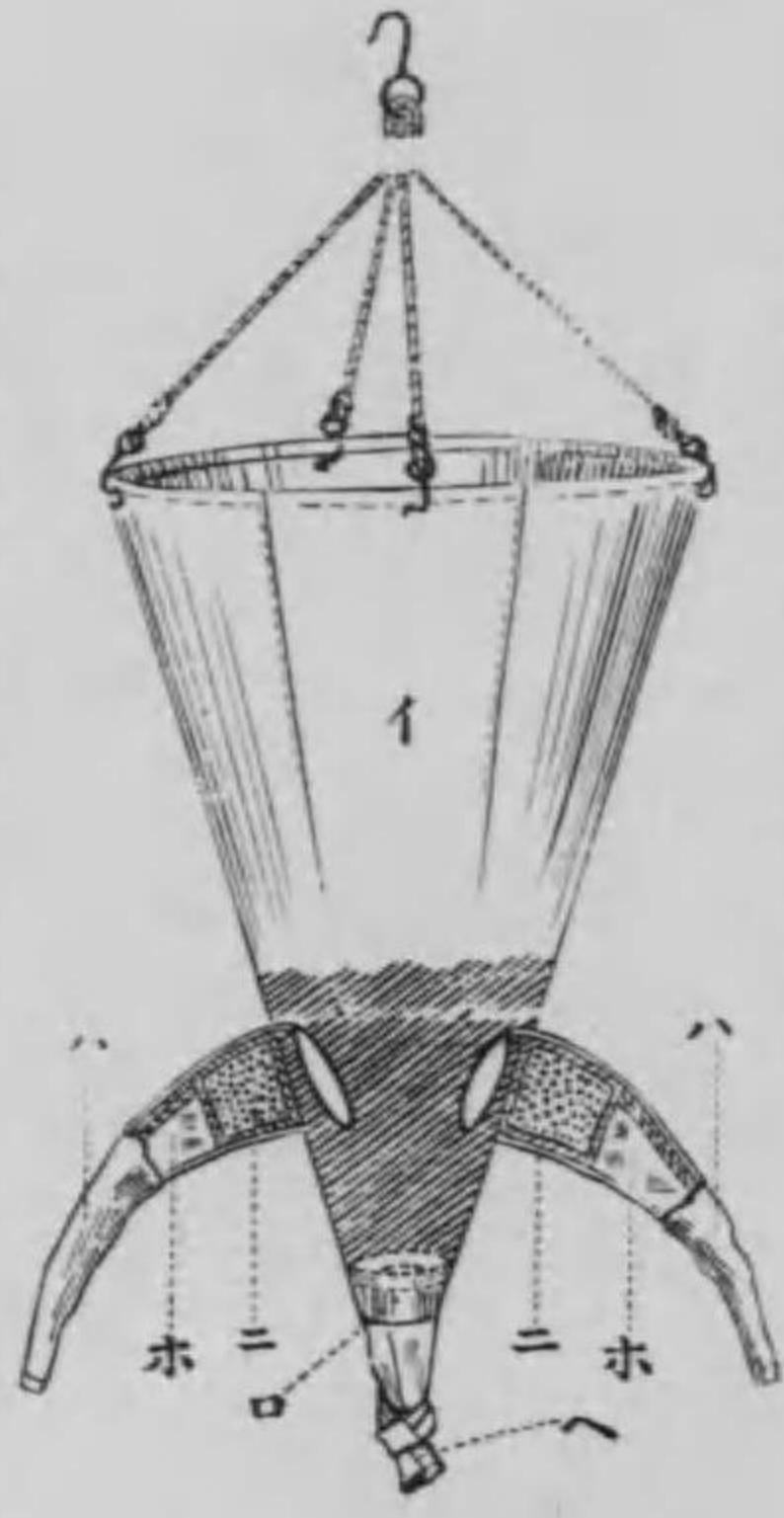
石地式濾過器 大、中型 流出口二箇所附
