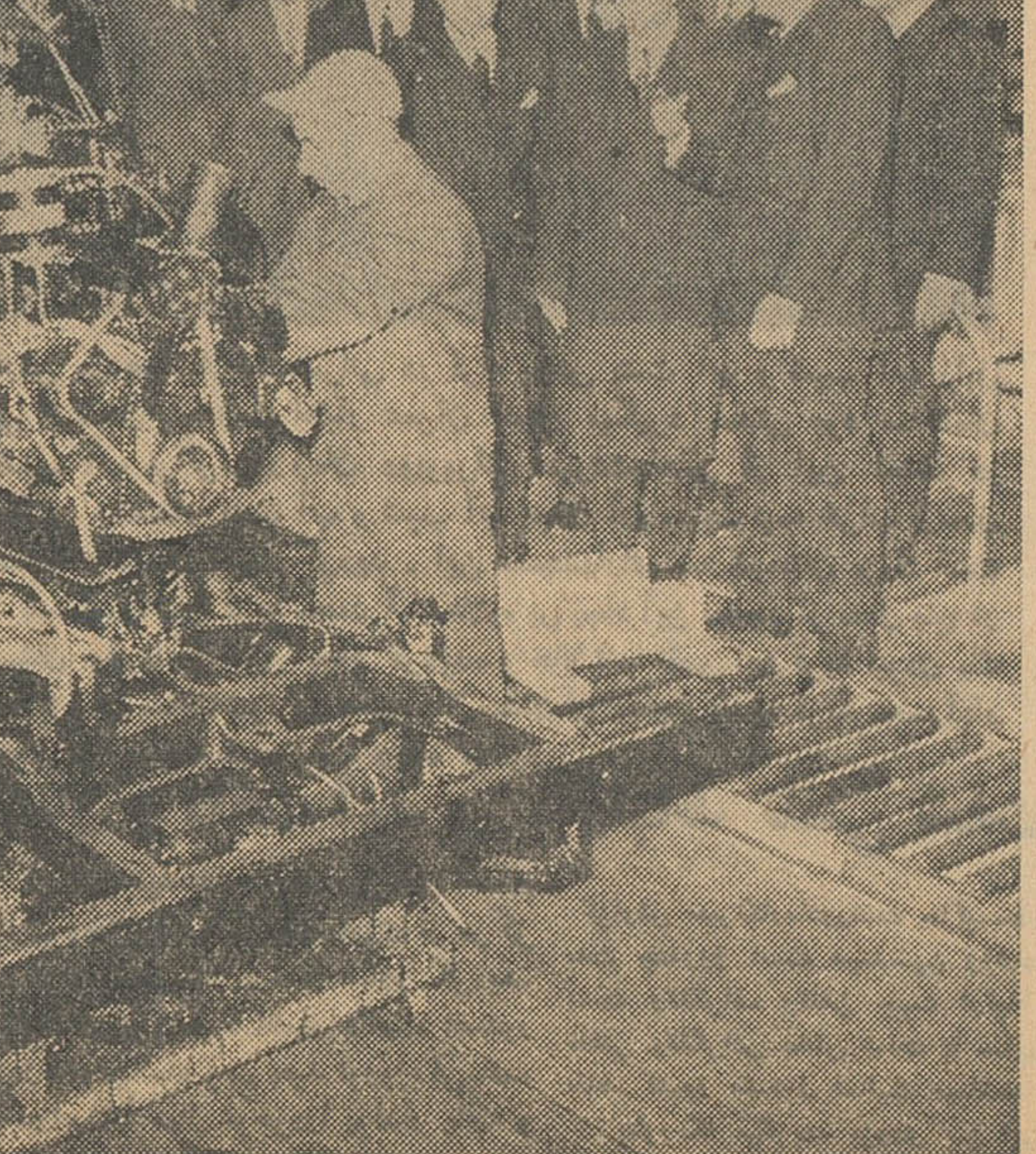
کارگران موتور رابرووی شاسی سوار میکنند
