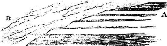
Fig. 2.—At the Embouchure of the Poulidu.
