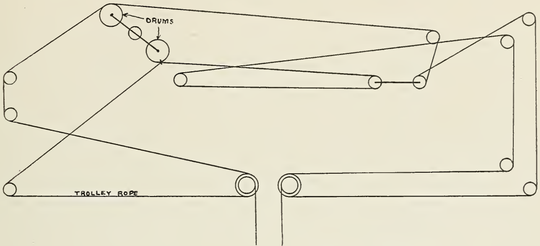
ORE UNLOADER RIG
