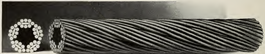
Type C—5 Strands 9 Wires—1 Hemp Core
