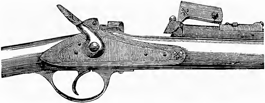
The Braendlin-Albini.
