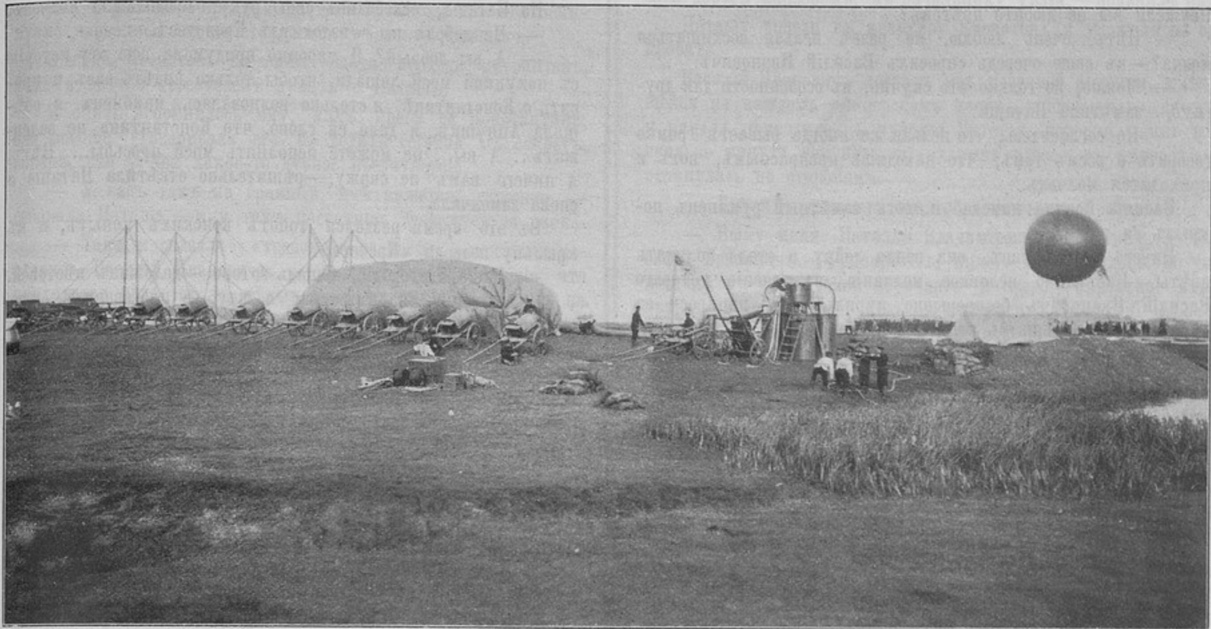
Воздухоплавательный паркъ. Лабораторія. Добываніе водорода и наполненіе шара газомъ (къ статьѣ «Курскіе маневры»).
