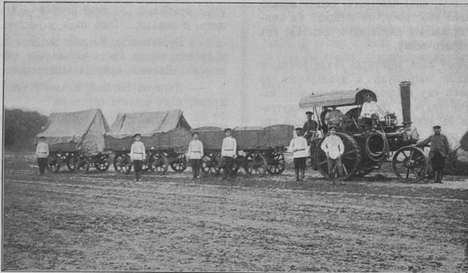
Дорожные паровозы въ Сѣверной арміи (къ статьѣ «Курскіе маневры»).
