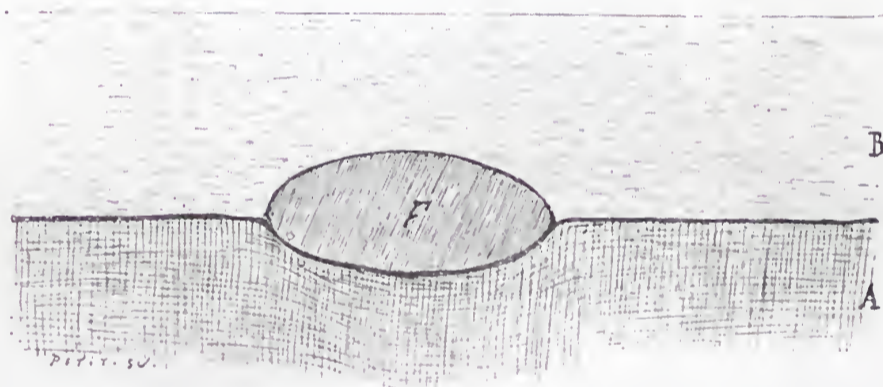
Fig. 2. — Corps organisé F comprimé par le poids de l'assise B nouvellement déposée, imprimant le moule de sa face inférieure à la superficie de l'assise inférieure A.
