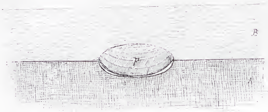
Fig. 3. — Corps organisé F graduellement décomposé, s'affaisant sous le poids de l'assise B dont le sédiment pénètre peu à peu dans la cavité résultant de cette décomposition.
