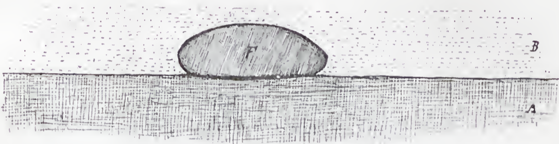
Fig. 1. — Corps organisé F couché sur le sol sous-marin, à la superficie d'une assise inférieure A, et recouvert par le sable d'une assise en voie de formation B.
