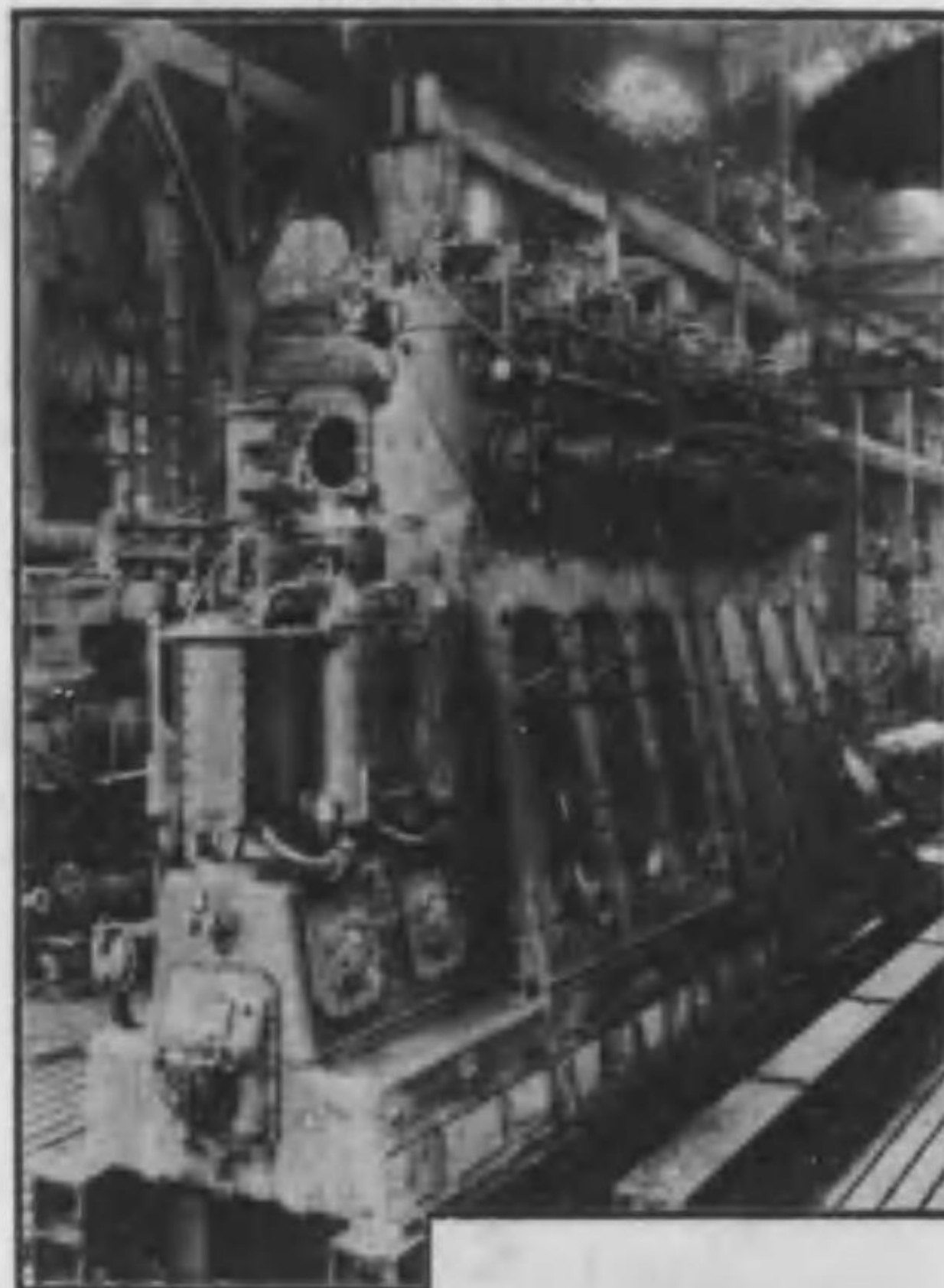
三菱ズルツアー式ディーゼルエンジン(二、三〇〇馬力) (長崎造船所製作)
