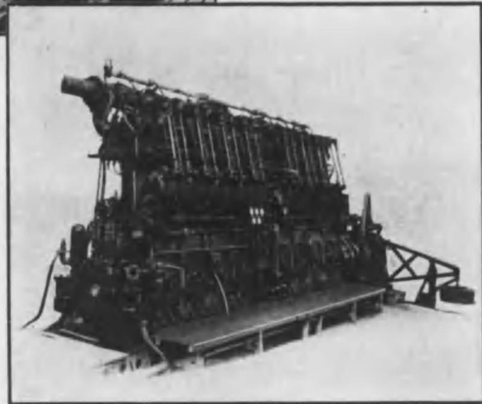
三菱ウイツカース式 ディーゼルエンジン(九二〇馬力) (神戸造船所製作)
