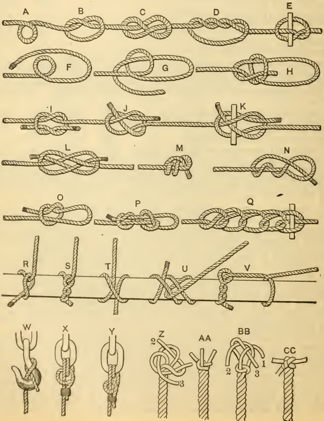
FIG. 95. — KNOTS.
