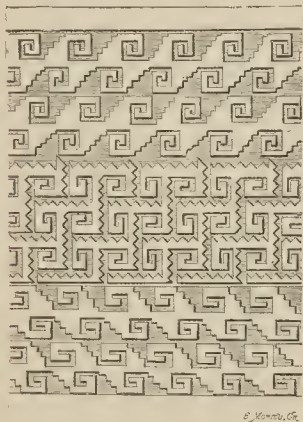
Fig. 2. - Mosaico que forma el revestimiento de todas las paredes de la cripta subterránea.
