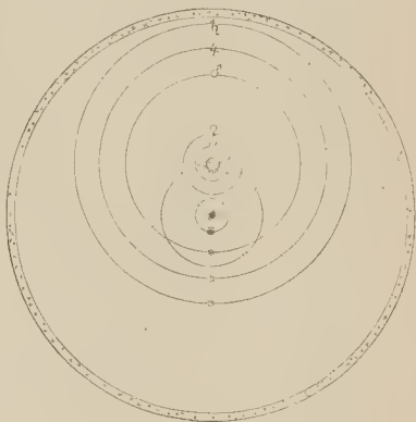
EL SISTEMA SOLAR DE TYCHO BRAHE
