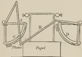
Fig. 1. - Aparato transmisor
