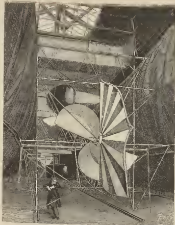
Fig. 3. - Vista de la parte posterior de la barquilla, con el timón, la hélice y el paracaídas
