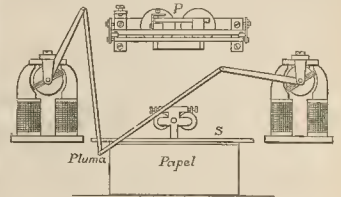
Fig. 4. - Aparato receptor
