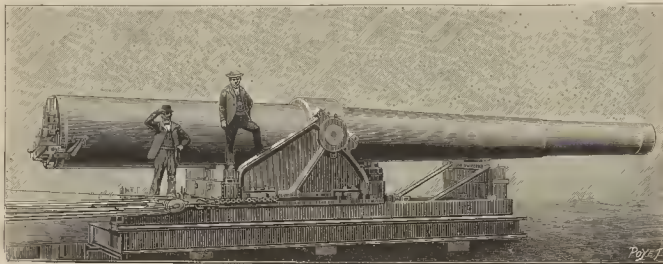
EL NUEVO CAÑÓN AMERICANO GATHMAN. - 1. Vista del cañón en conjunto
