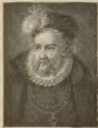
EL ASTRÓNOMO TYCHO BRAHE
