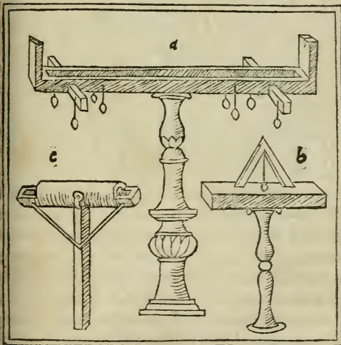
a. chorobates
