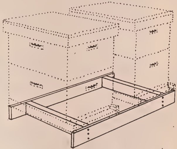
Double hive-stand.
