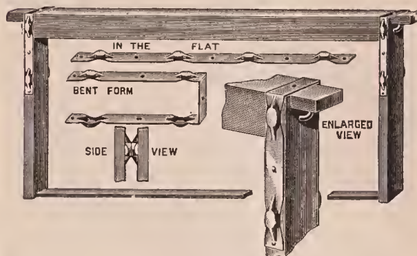
Metal-space Hoffman frame.
