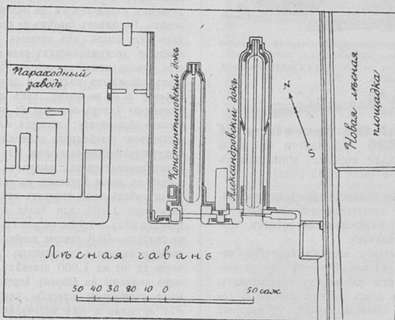
Чертежъ вновь открытаго Александровскаго дона въ Кронштадтѣ (см. корреспонд. «Кронштадтъ» на стр. 1009).
