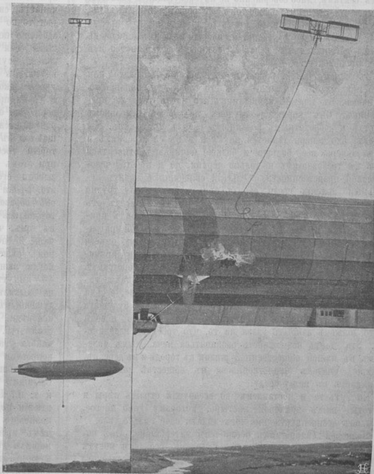
Предлагаемый полковникомъ англійской службы Ноди новый способъ борьбы аэроплановъ съ воздушными кораблями. Аэропланъ ловитъ корабль на „удочку“, снабженную бомбой.
