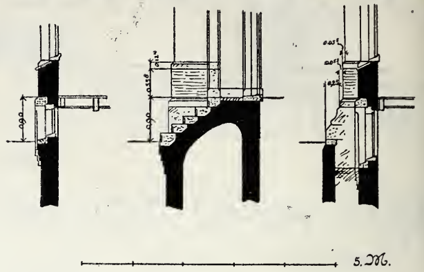
Doorsn: C-D Doorsn: E-H Doorsn: A-B
