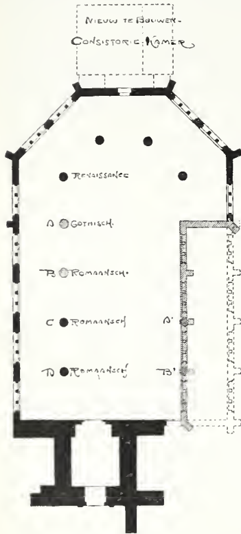
Plattegrond. Schaal 1 à 400.
