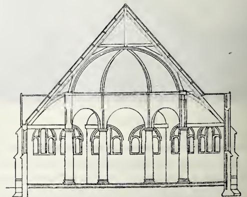
Doorsnede over de breedte. Schaal 1 à 300.
