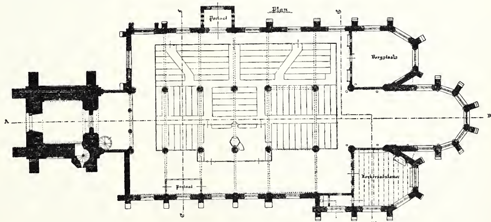
Plattegrond. Schaal 1 à 500.
