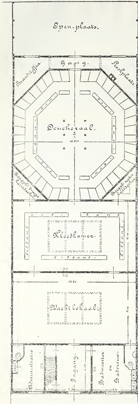
Plattegrond. Schaal 1 à 200.
