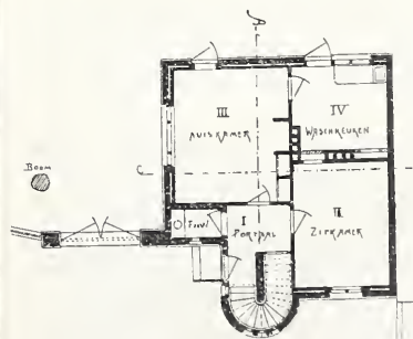
Beganegrond *) schaal 1 à 300.
