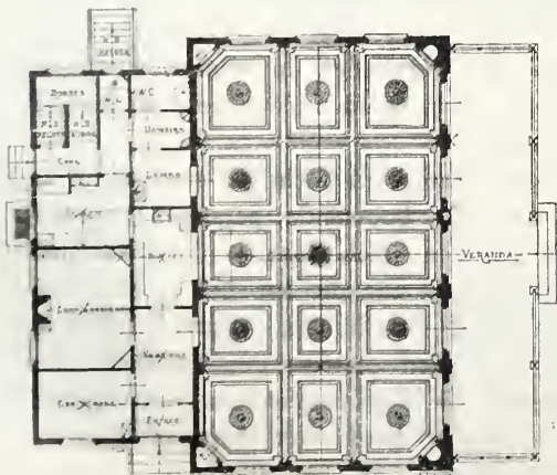
Beganegrond. Schaal 1 à 300.
