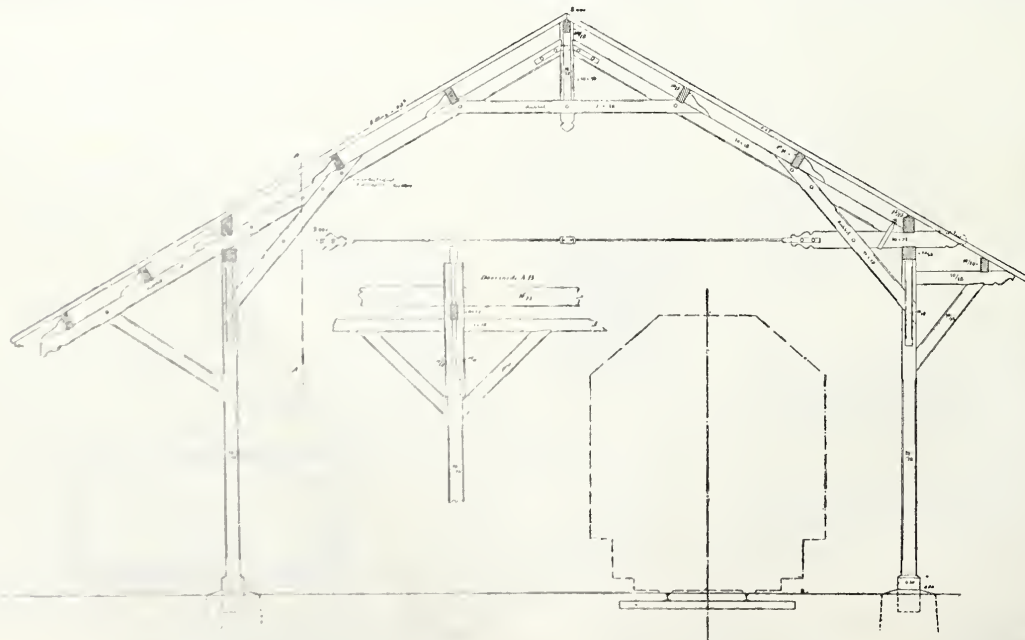
Type van een Stationskap. Schaal 1 à 100.
