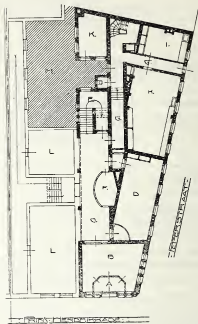
Plan beganegrond. Schaal 1 à 400.
