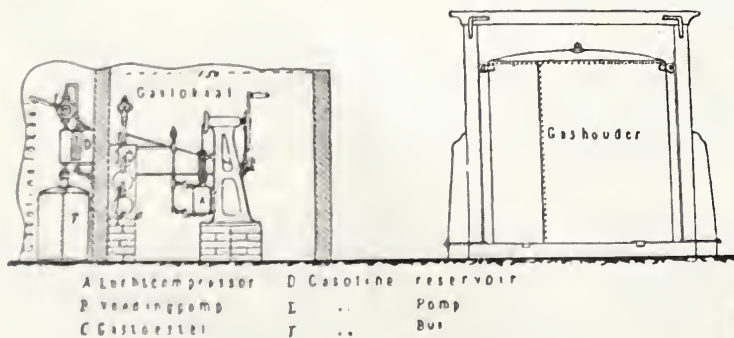
Fig. 1 stelt eene luchtgasinrichting voor met eene gasproductie van 7500 liter per uur. Zij bestaat uit: A, een toestel voor het afmeten en samenpersen der benodigde
