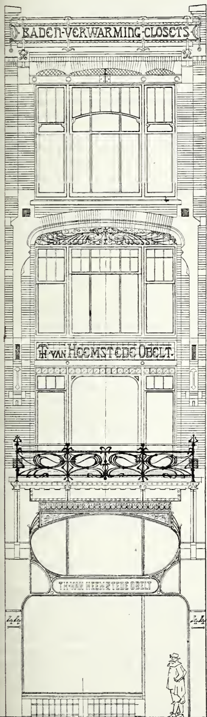
Magazijn aan het Rokin te Amsterdam. Schaal 1 à 100.
