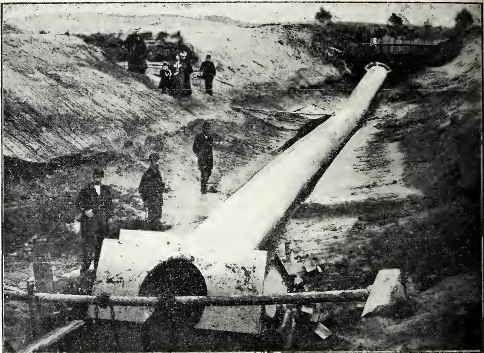
Duiker van 1 M. middellijn en 36 M. lengte, gemaakt in September 1896 onder de Schaapshokswijk te Veenhuizen, ten behoeve van den Rijkswaterstaat.
