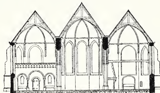
Dwarsdoorsnede over CD. Schaal 1 à 400.
