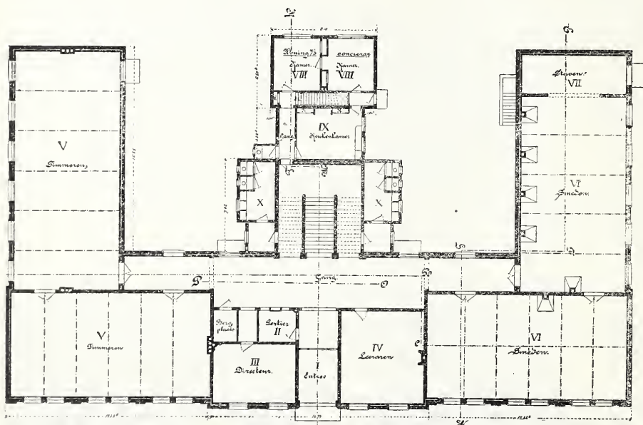
Begane grond. Schaal 1 à 400.
