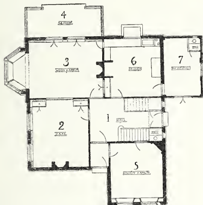
Beganegrond. Schaal 1 à 300.
