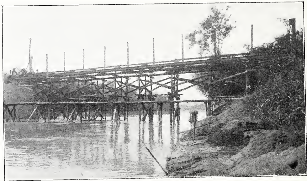
Monteeren van een brug van 40 M. spanning.
