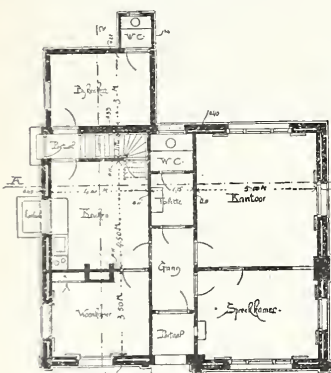
Beganegrond. Schaal 1 à 300.
