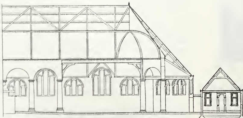
Doorsnede over de lengte. Schaal 1 à 300.
