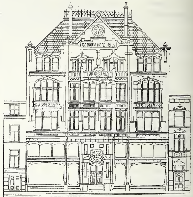
Voorgevel, Schaal 1 à 300.
