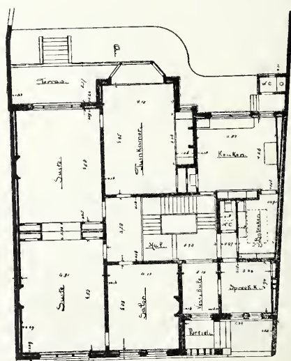
Begane grond. Schaal 1 à 300.
