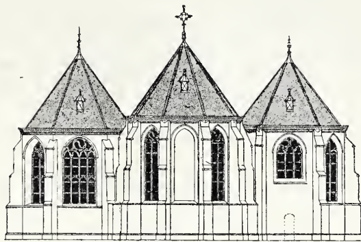
Oostelijke gevel. Schaal 1 à 300.
