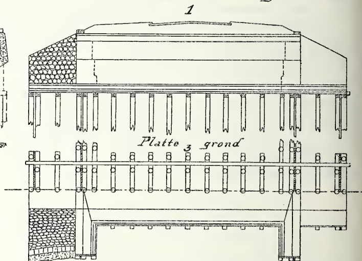
Gemetselde duiker. Schaal 1 à 200.
