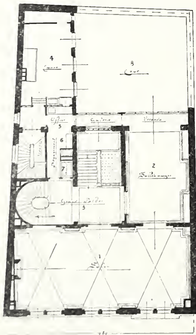
Hotel 8 Rue de Lota. Eerste verdieping. Schaal 1 à 300.
