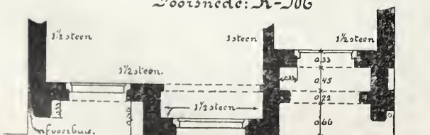
Doorsnede: K-M
