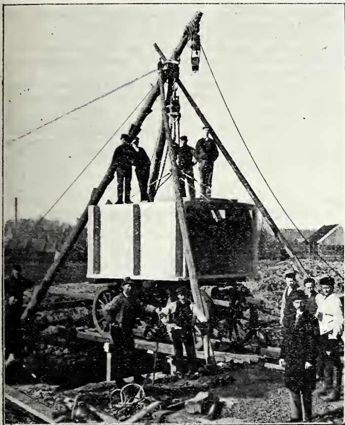
Twee duikers voor de Erven EKKER te Hengelo in de Diemerbeek, elk lang 69 M., breed 2.25 M., hoog 1.50 M., bestand tegen raddrukken van 3000 KG.
