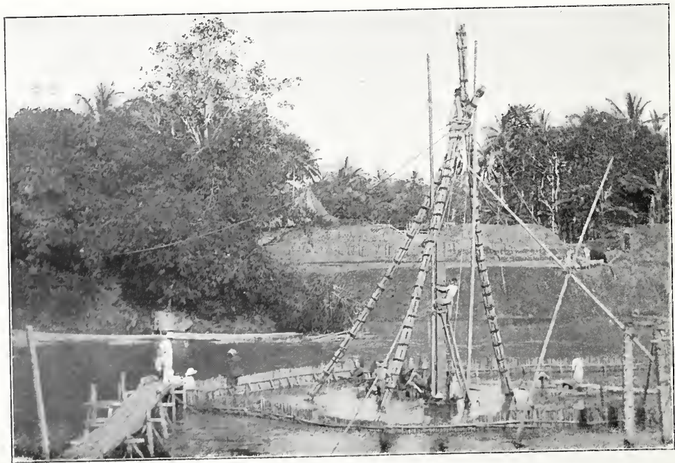
Het heien der eerste hoekpalen.
