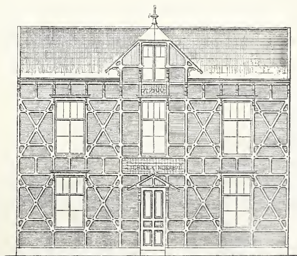
Voorgevel. Schaal 1 à 150.
