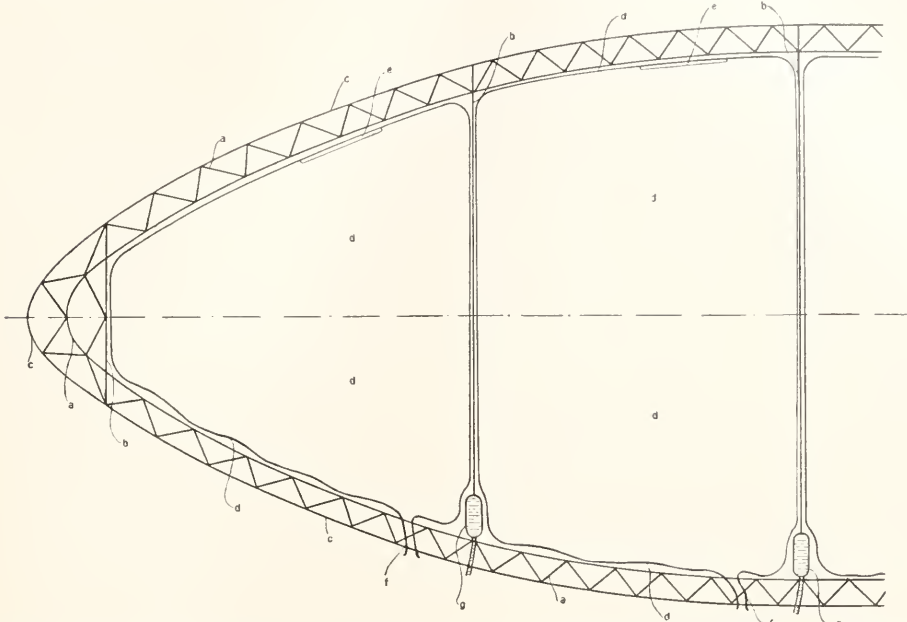
Fig. 4. Zeppelin-Lenkballon, Vorderteil. a Aluminiumgerüst, b Versteifungsringe, c äußere Hülle, d Hülle der Gasbehälter, e Ballonventile, f Füllansätze, g Wasserballastsäcke mit Abflußschläuchen.
