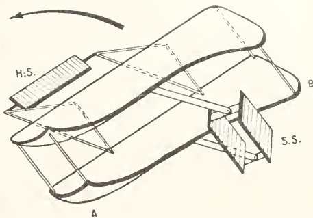
Fig. 11. Erklärung des Kurvenfluges durch die Quersteuerung am Wright-Apparat. Tragflächeneseite A hoch gebogen (sinkt deshalb), B nach unten gebogen (wird daher angehoben). Seitensteuer SS nach rechts ausgelegt, Höhensteuer HS aufwärts gestellt.
