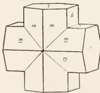
Fig. 23. Staurolith. Prisma m = \{110\} , \infty P ; seitliche Endfläche b = \{010\} , \infty P \infty ; Basis c = \{001\} , \infty P . Durchkreuzungszwilling nach dem Brachydoma \{032\} ; \frac{3}{2}P \infty .
