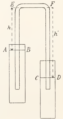
Fig. 4. Heber.
