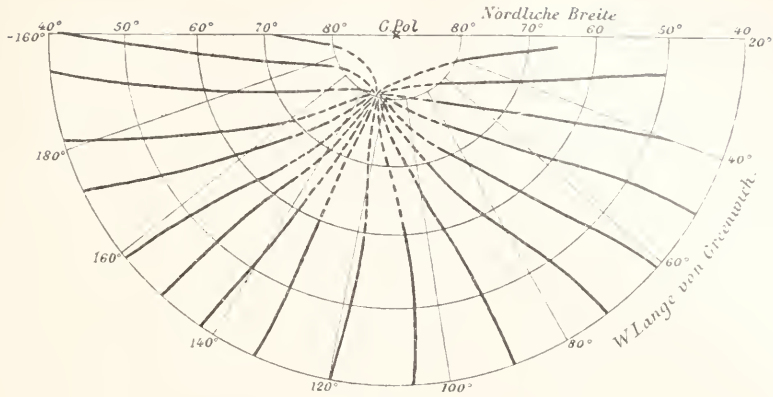
Magnetische Meridiane für 1600.
