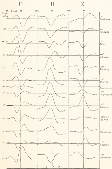
Fig. 5. Tägliche Variation der erdmagnetischen Elemente zur Äquinoktialzeit ( 1^{mm} = 6\gamma ).
