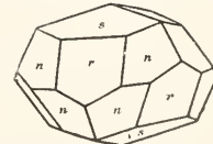
Fig. 30. Häematit.
