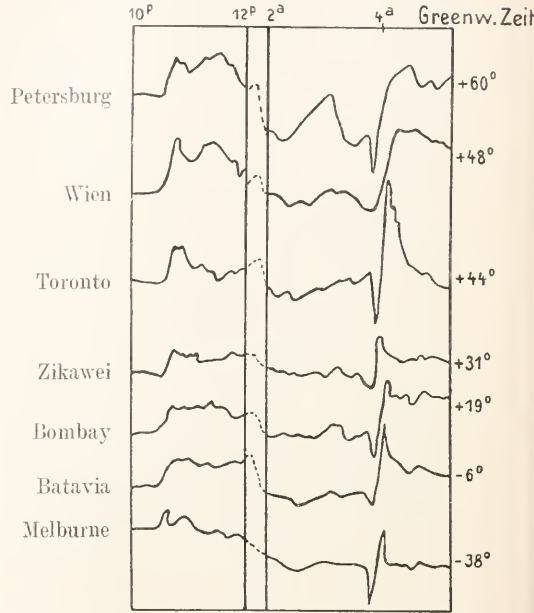
Fig. 19. Erdmagnetische Störung vom 24.—25. Juli 1885. Amplitude in Toronto 470γ, in Wien 120γ (Maßstab bei den einzelnen Stationen verschieden).
