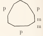
Fig. 15b. Turmalin-Querschnitt.
