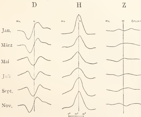
Fig. 6. Täglicher Gang der erdmagnetischen Elemente in Apia, Samoa ( 1^{mm} = 6\gamma ).
