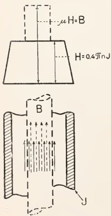
Fig. 2. Magnetisches Feld einer unendlich (oder) langen Spule.
