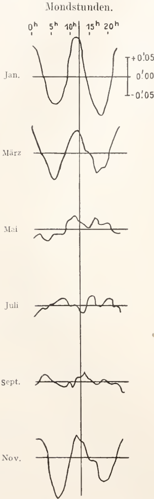
Fig. 16. Mondtägliche Aenderung der Dekl. in Batavia im Laufe des Jahres 1 mm = 0'.01.
