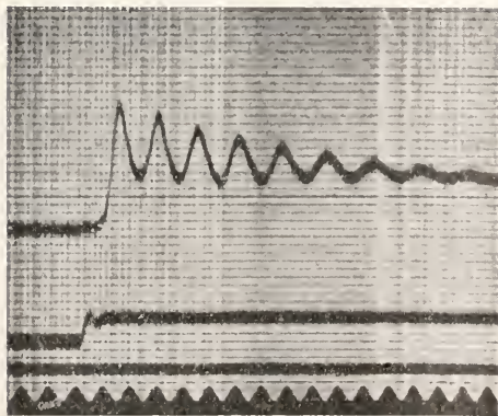
Fig. 14. Rhythmische Aktionsstörung bei Reizung des Schildkrötenmuskels mit dem konstanten Strom. Nach Dittler und Oinuma.
