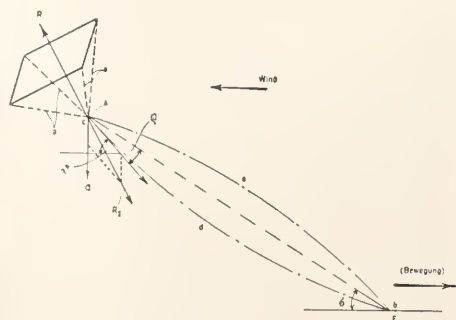
Fig. 7. Schema des Drachen. A Befestigungspunkt der Last Q, E Haltepunkt am Erdboden, a Schnüre zur Einstellung des richtigen Winkels (der Bucht), Wkl. \sigma \sim Wkl. \rho , daraus zu berechnen, bdc Krümmung der Leine, bec Weg des Drachens beim Aufstieg.
