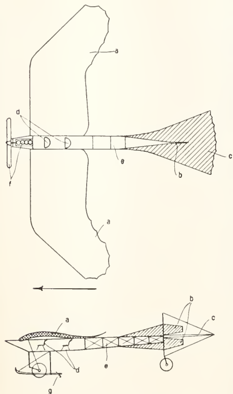
Fig.15. Etrich-Rumpler-Eindecker. a Tragfläche, b Seitensteuer, c Höhensteuer, d Sitze, e Gestell, f Motor und Propeller, g Bremssporn beim Landen.
