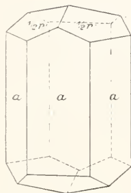
Fig. 2 bis 4. Kalkspat.
