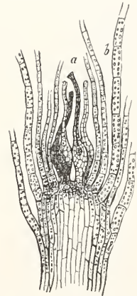
Fig. 20. Archegonienstand eines Moores. a Archegonien, b Hüllblätter. Nach Goebel.
