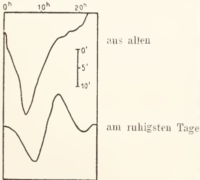
Fig. 13b. Deklination Mai 1910. Dyraifjord, Island.
