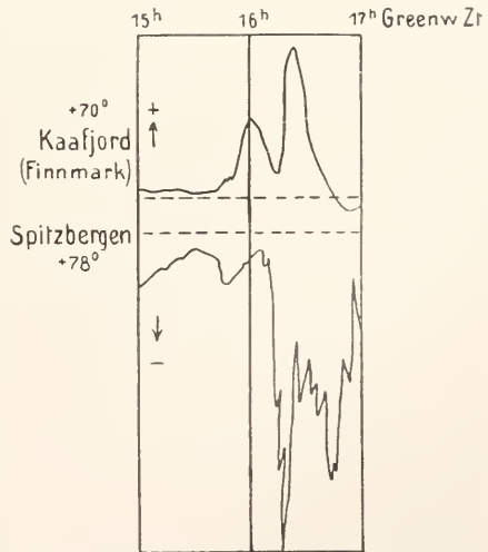
Fig. 22. Horizontale Intensität der Störung vom 15. II. 1903. 1 mm = 10γ. Entfernung Kaafjord — Spitzbergen = 900 km.
