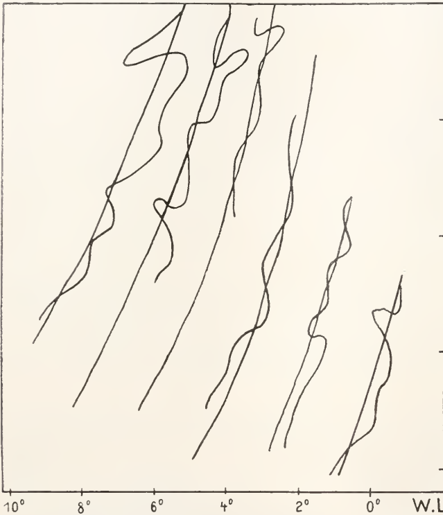
Fig. 3. Terrestrische und wahre Isogonen in Großbritannien.
