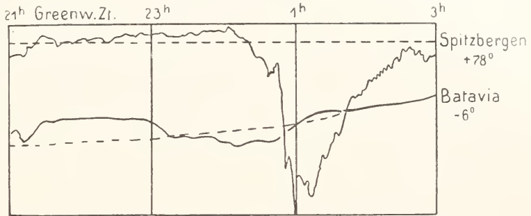
Fig. 21. Horizontale Intensität der Störung vom 31. März 1903. 1 mm = 3.5γ nach oben wachsend. 21h—23h Äquatoriale, 0h—3h polare Störung — — — — normaler tägl. Gang.
