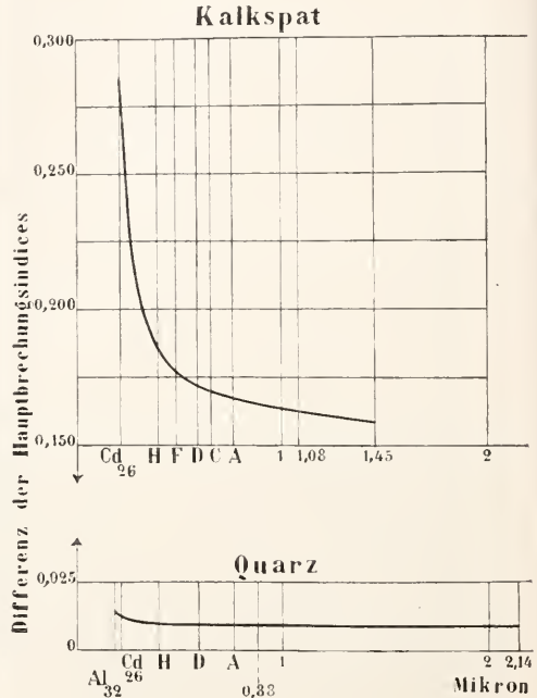
Fig. 10. Dispersion der Doppelbrechung.
