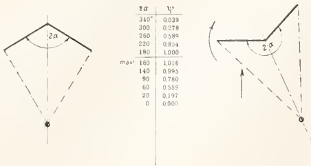
Fig. 8. Fallschirm. Ist 2\alpha der Spitzwinkel, so ist die Tragkraft k = \psi \cdot k_e , wenn k_e = Tragkraft der gleich großen ebenen Fläche ist.
